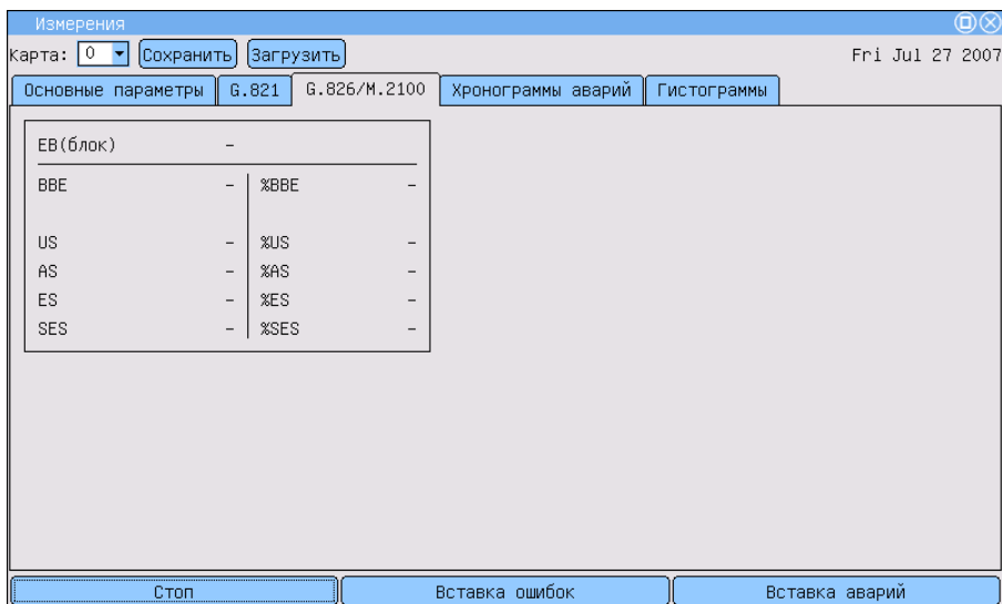
Рис. 4.3: Измерения. ITU-T G.826/М.2100
