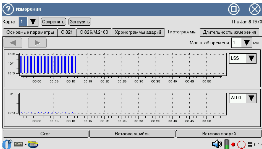
Рис. 5.1: Гистограммы аварий и ошибок
