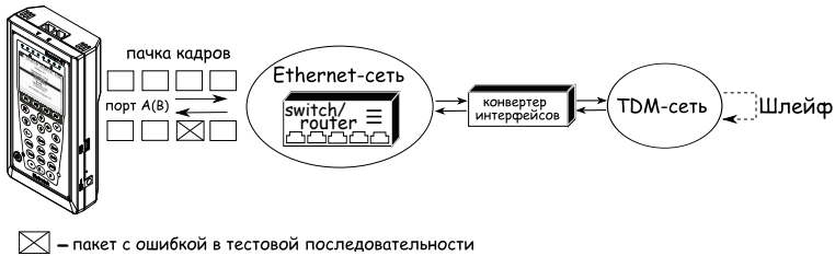
Рис. 7.56. Тестирование на канальном/сетевом уровне (вариант 1)
