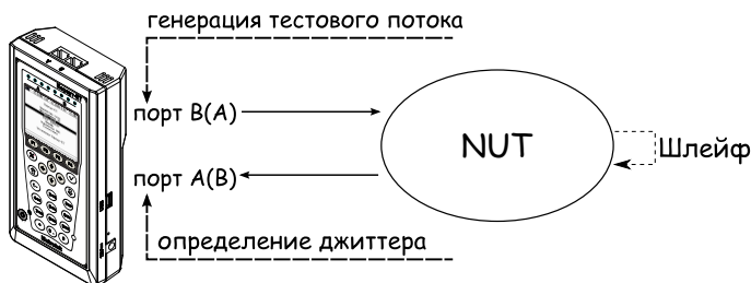
Рис. 7.62. Измерение джиттера. Схема 1
