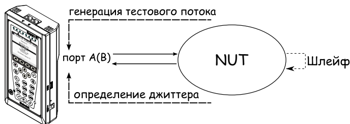
Рис. 7.64. Измерение джиттера. Схема 3
