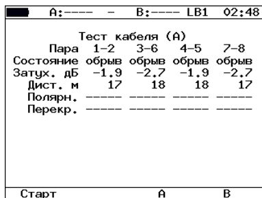
Рис. 7.47. Экран «Тест кабеля»
