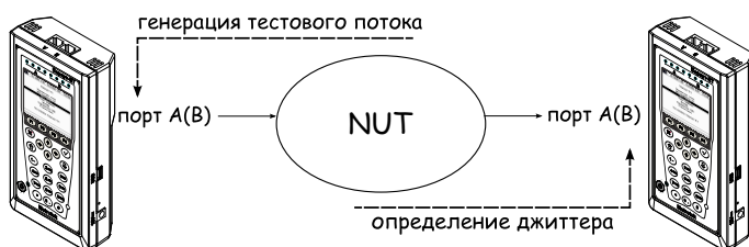
Рис. 7.63. Измерение джиттера. Схема 2
