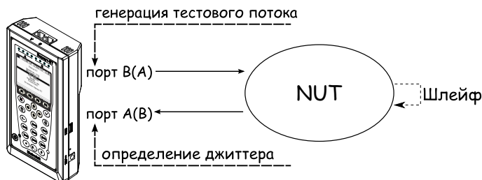
Рис. 7.62. Измерение джиттера. Схема 1
