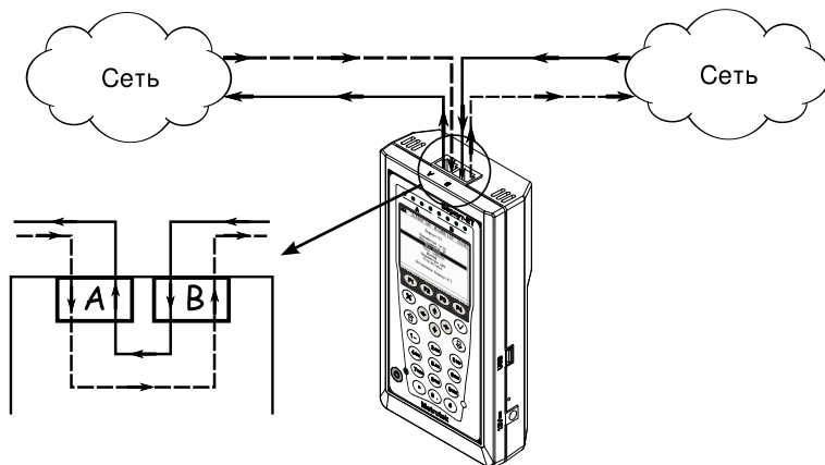
Рис. 7.45. Пример подключения в режиме «Транзит»
