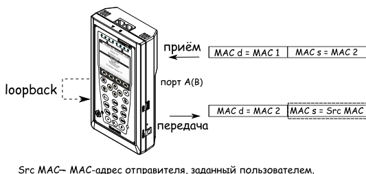
Рис. 7.28. Режим замены «Отпр.»
