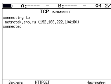
Рис. 7.42. Пример успешного соединения с узлом
