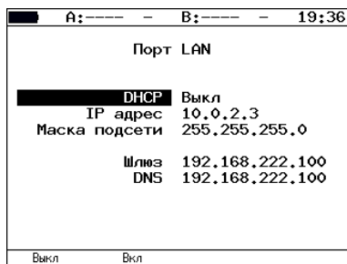
Рис. 7.78. Меню «Порт LAN»
