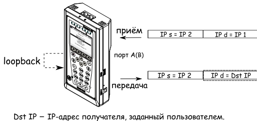
Рис. 7.32. Режим замены «Получ.»
