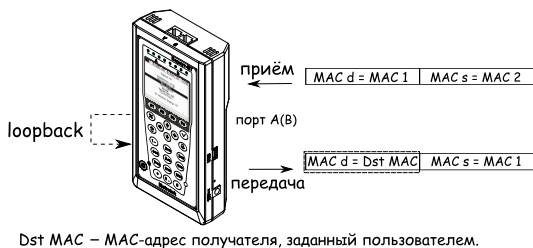
Рис. 7.27. Режим замены «Получ.»
