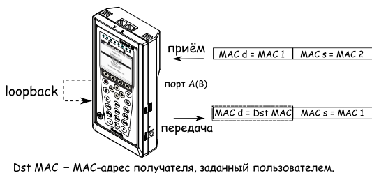
Рис. 7.40. Режим замены «Получ.»
