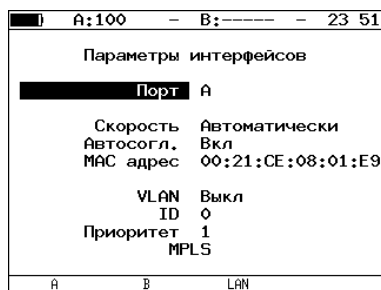
Рис. 7.96. Меню «Параметры интерфейсов»
