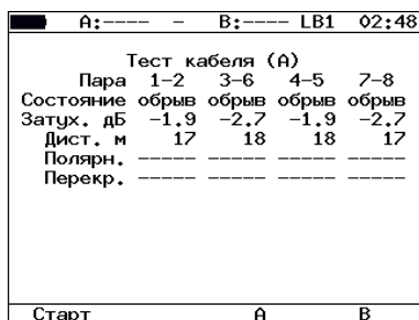
Рис. 7.64. Экран «Тест кабеля»
