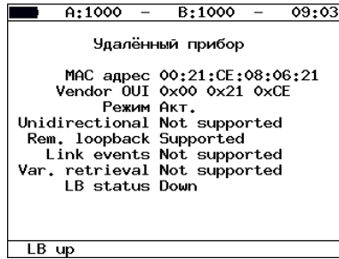
Рис. 7.49. Экран «Удалённый прибор»
