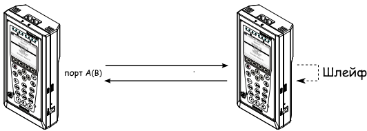
Рис. 7.75. Тестирование на физическом уровне (вариант 2)
