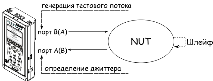
Рис. 7.84. Измерение джиттера. Схема 2
