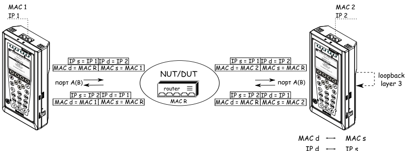
Рис. 7.6. Вариант подключения 2
