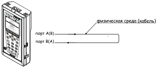
Рис. 7.74. Тестирование на физическом уровне (вариант 1)
