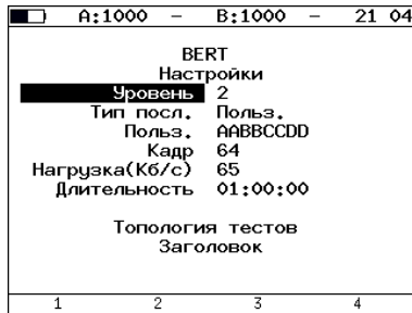
Рис. 7.70. Меню «Настройки BERT»
