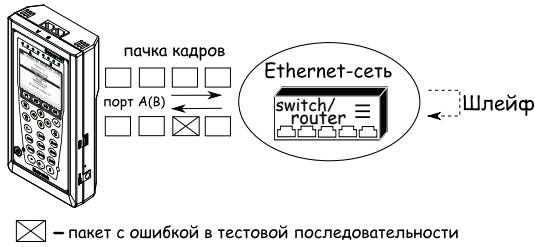
Рис. 7.77. Тестирование на канальном/сетевом уровне (вариант 2)
