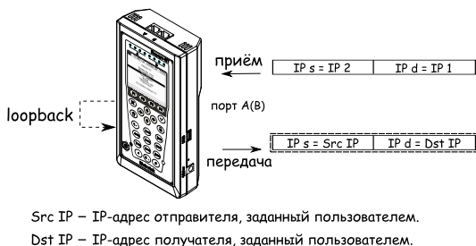
Рис. 7.46. Режим замены «Оба»
