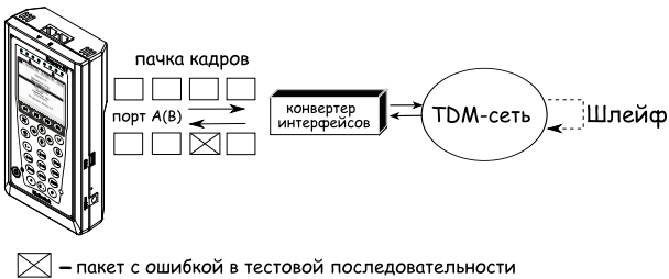
Рис. 7.78. Тестирование на канальном/сетевом уровне (вариант 3)
