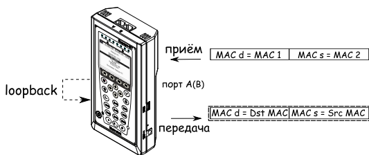
Рис. 7.42. Режим замены «Оба»
