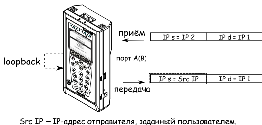
Рис. 7.44. Режим замены «Отпр.»
