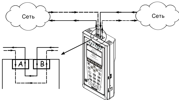
Рис. 7.62. Пример подключения в режиме «Транзит»
