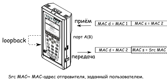
Рис. 7.41. Режим замены «Отпр.»
