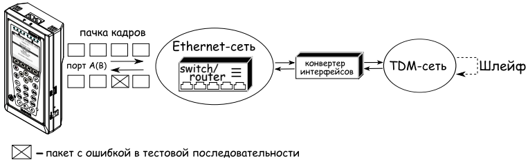
Рис. 7.76. Тестирование на канальном/сетевом уровне (вариант 1)
