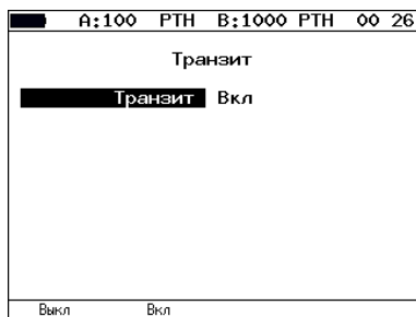
Рис. 7.73. Меню «Транзит»
