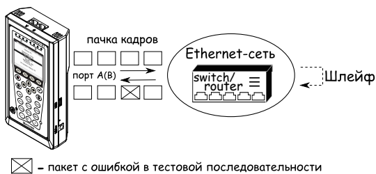
Рис. 7.88. Тестирование на канальном/сетевом уровне (вариант 2)
