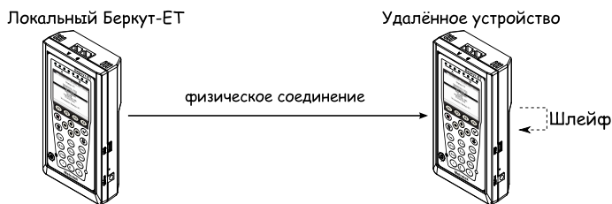
Рис. 7.51. Схема тестирования
