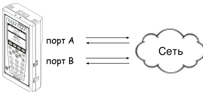
Рис. 7.58. Вариант подключения 2
