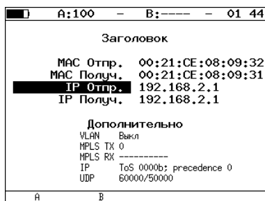
Рис. 7.10. Меню «Заголовок»
