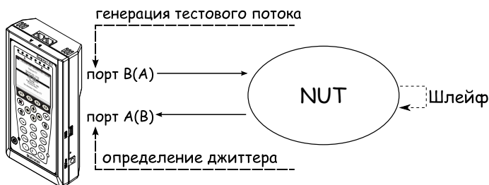
Рис. 7.95. Измерение джиттера. Схема 2
