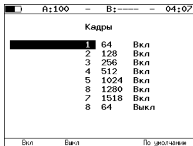
Рис. 7.15. Меню «Кадры»
