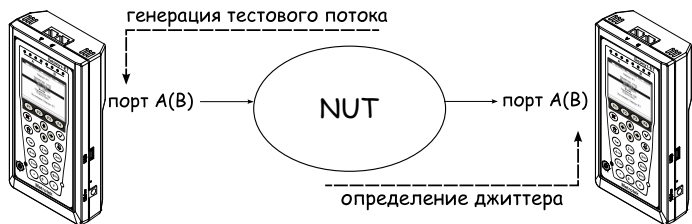
Рис. 7.99. Измерение джиттера. Схема 3
