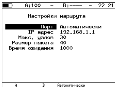
Рис. 7.67. Меню «Настройки маршрута»
