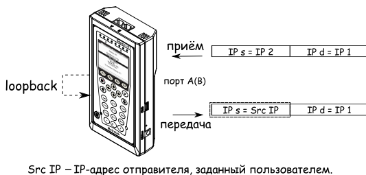
Рис. 7.51. Режим замены «Отпр.»
