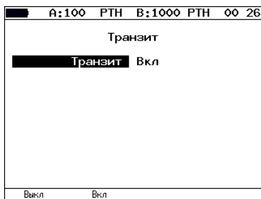
Рис. 7.76. Меню «Транзит»
