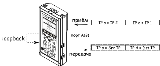
Рис. 7.53. Режим замены «Оба»
