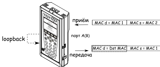
Рис. 7.47. Режим замены «Получ.»
