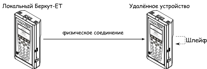
Рис. 7.54. Схема тестирования
