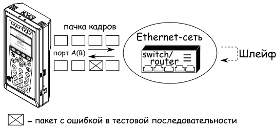
Рис. 7.91. Тестирование на канальном/сетевом уровне (вариант 2)
