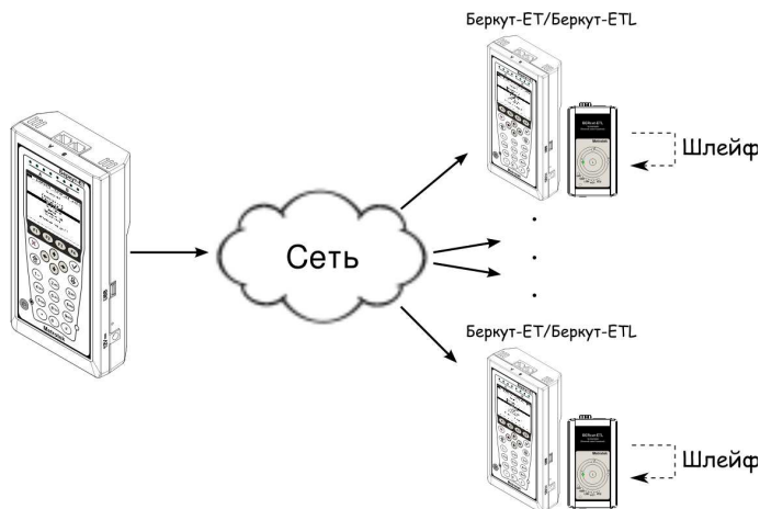
Рис. 7.57. Схема тестирования
