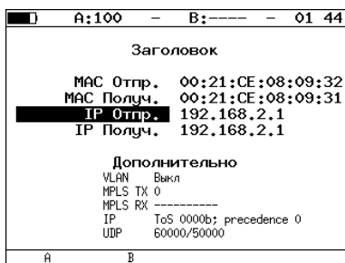
Рис. 7.13. Меню «Заголовок»
