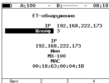
Рис. 7.59. Пример выполнения E-T-обнаружения
