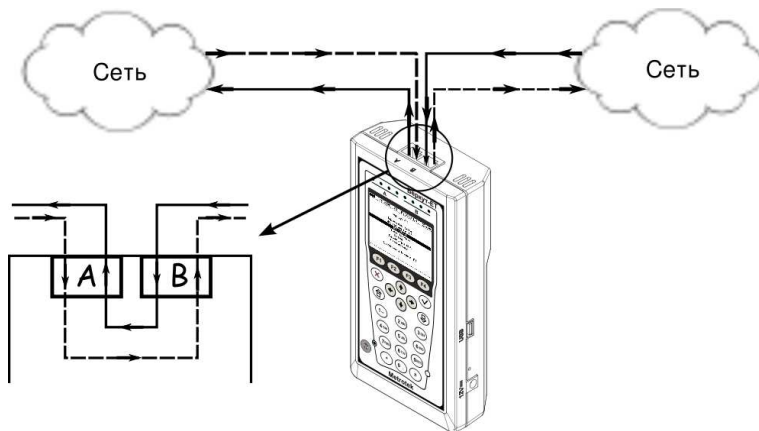
Рис. 7.75. Пример подключения в режиме «Транзит»
