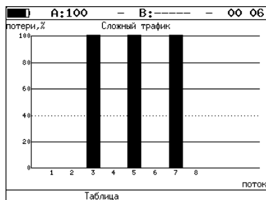
Рис. 7.36. Экран «Сложный трафик» (график)
