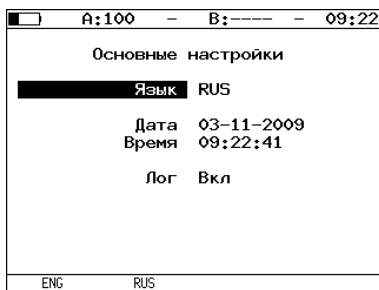
Рис. 7.116. Меню «Основные настройки»
