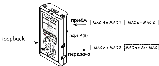
Рис. 7.48. Режим замены «Отпр.»
