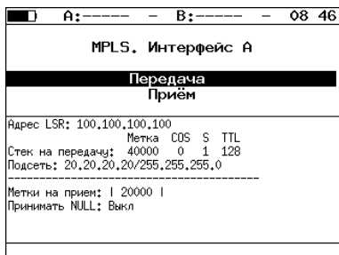
Рис. 7.111. Меню «MPLS. Интерфейс А»
