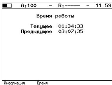
Рис. 7.118. Экран «Время работы»
