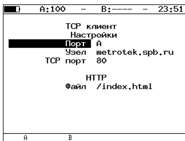
Рис. 7.72. Настройки теста «TCP-клиент»
