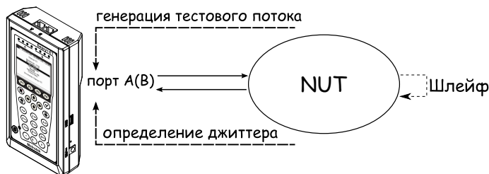
Рис. 7.97. Измерение джиттера. Схема 1
