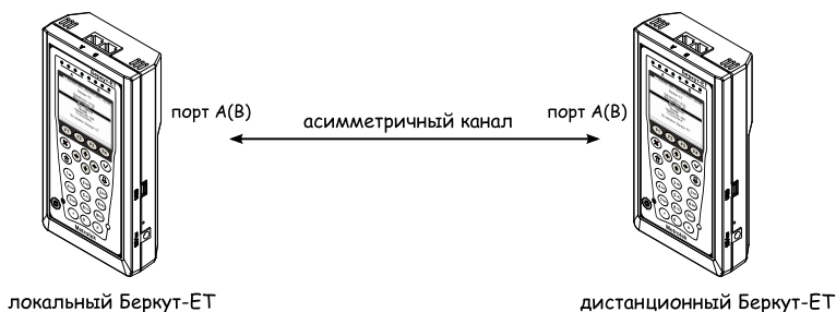
Рис. 7.33. Схема подключения
