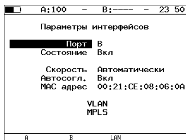
Рис. 7.110. Меню «Параметры интерфейсов»
