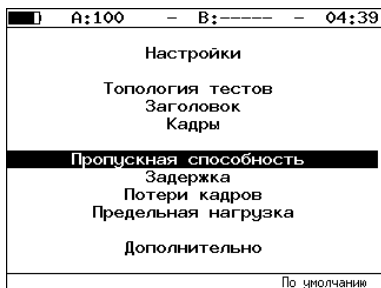
Рис. 7.12. RFC 2544. Настройки
