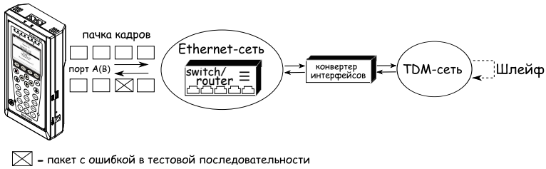
Рис. 7.90. Тестирование на канальном/сетевом уровне (вариант 1)
