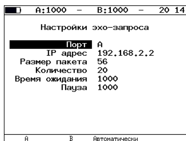
Рис. 7.63. Меню «Настройки эхо-запроса»
