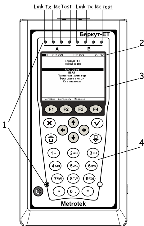
Рис. 6.1. Лицевая панель
