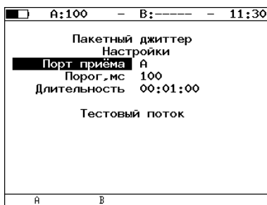
Рис. 7.96. Меню «Пакетный джиттер. Настройки»
