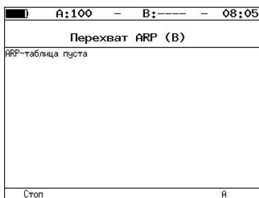
Рис. 7.70. Меню «Перехват ARP»
