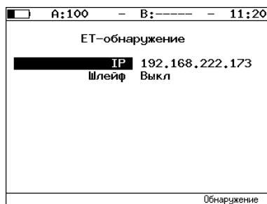
Рис. 7.58. Меню «ЕТ-обнаружение»
