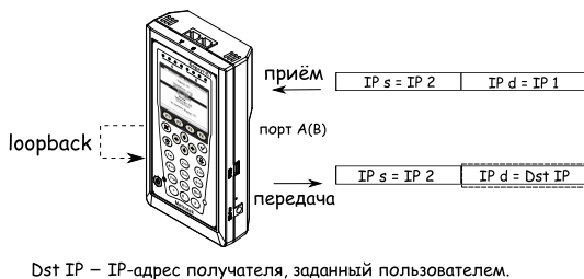
Рис. 7.52. Режим замены «Получ.»
