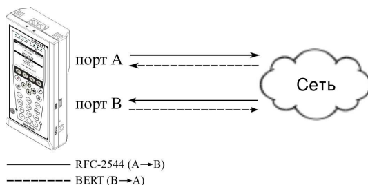
Рис. 7.9. Схема подключения
