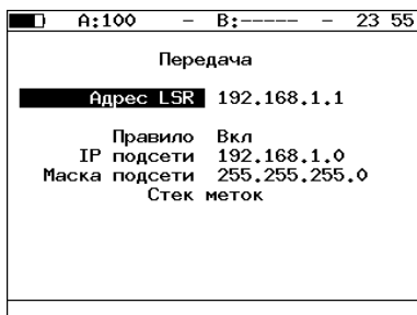
Рис. 7.112. Меню «Передача»
