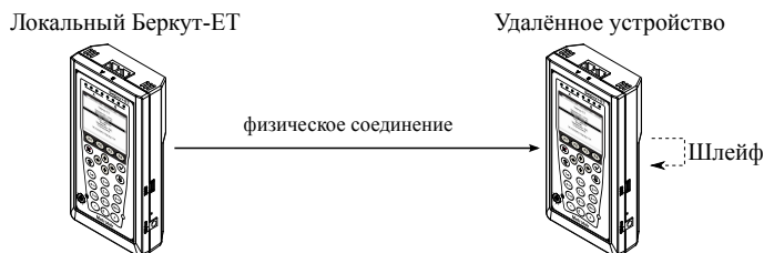
Рис. 7.59. Схема тестирования
