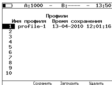
Рис. 7.126. Меню «Профили»
