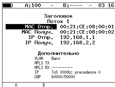
Рис. 7.46. Меню «Заголовок»
