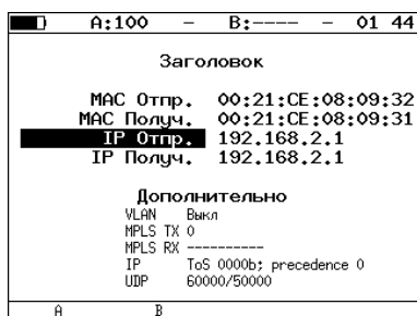
Рис. 7.13. Меню «Заголовок»
