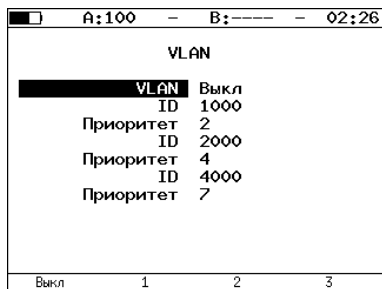
Рис. 7.15. Меню «VLAN»
