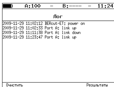
Рис. 7.128. Меню «Лог»
