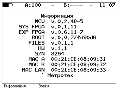
Рис. 7.122. Экран «Информация»
