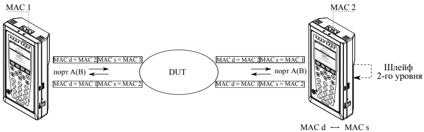
Рис. 7.5. Вариант подключения 1
