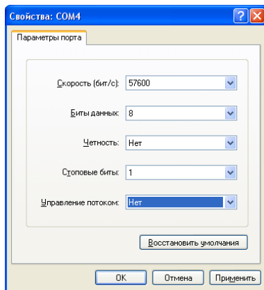
Рис. 8.4. Параметры порта
