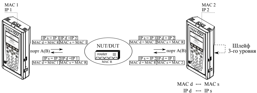
Рис. 7.6. Вариант подключения 2
