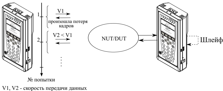
Рис. 7.1. Анализ пропускной способности
