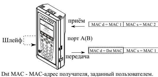
Рис. 7.52. Режим замены «Получ.»
