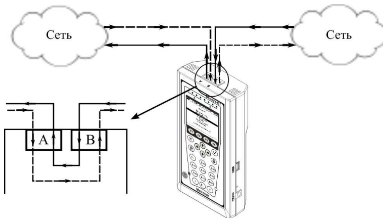
Рис. 7.80. Пример подключения в режиме «Транзит»
