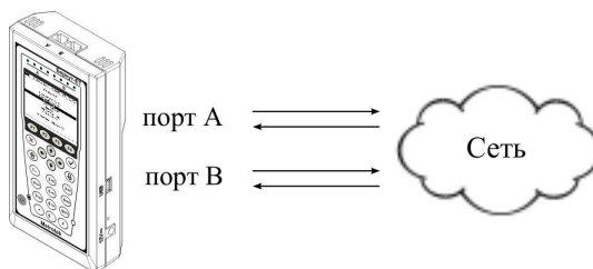
Рис. 7.66. Вариант подключения 2
