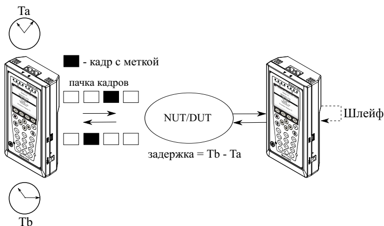
Рис. 7.2. Анализ задержки
