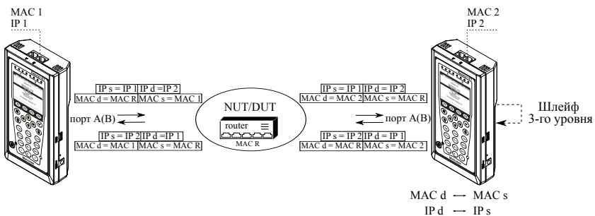
Рис. 7.6. Вариант подключения 2
