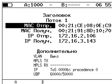
Рис. 7.36. Экран «Заголовок»
