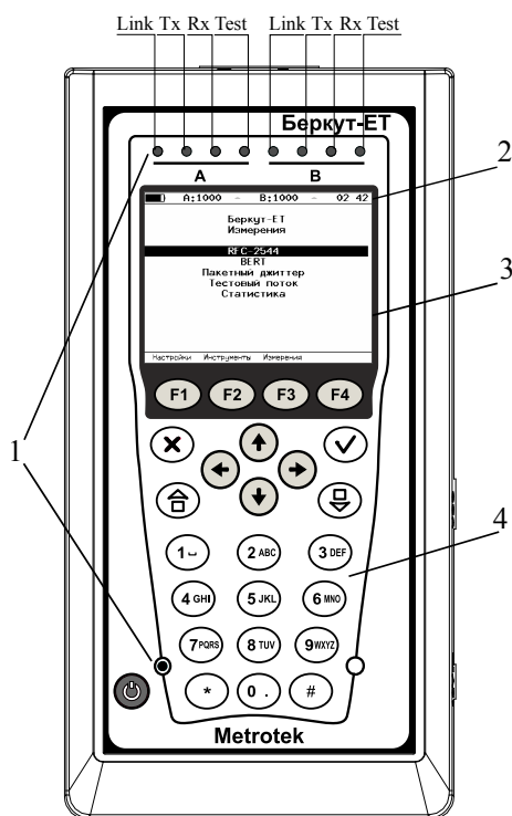
Рис. 6.1. Лицевая панель
