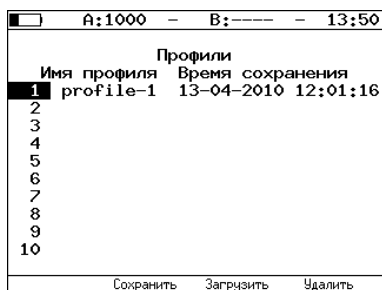
Рис. 7.126. Меню «Профили»
