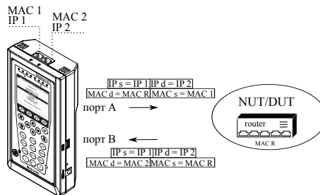
Рис. 7.7. Вариант подключения 3
