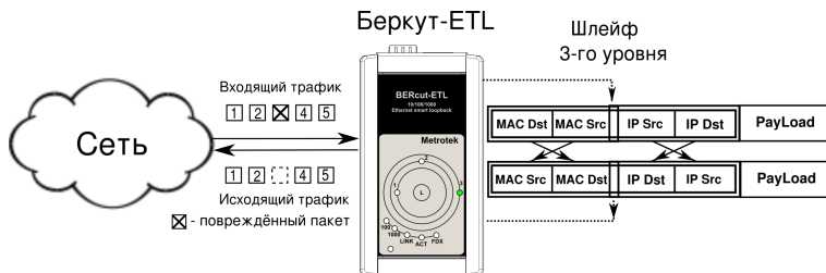
Рис. 4.3. Подключение шлейфа 3-го уровня
