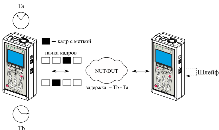
Рис. 5.2. Анализ задержки
