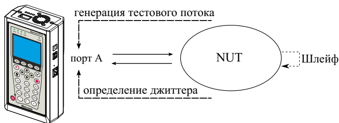
Рис. 14.5. Измерение джиттера. Схема 1
