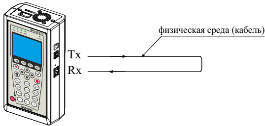
Рис. 13.8. Тестирование на физическом уровне (вариант 1)
