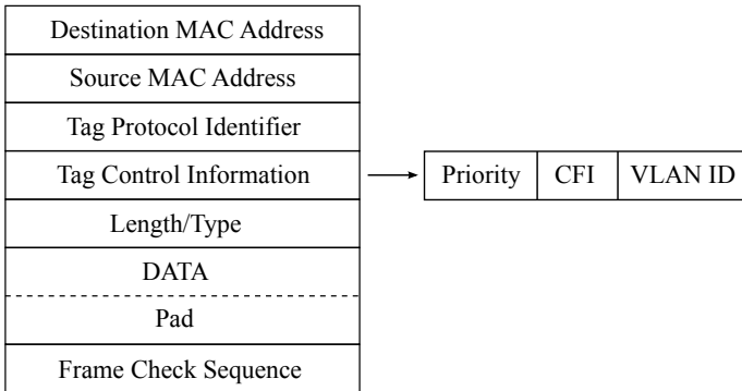
Рис. С.2. Структура Ethernet-кадра, содержащего VLAN-метку
