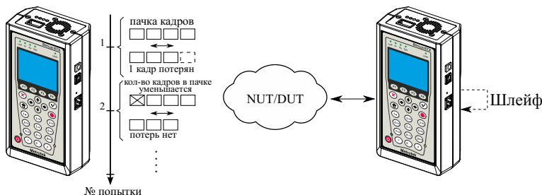
Рис. 5.4. Анализ предельной нагрузки
