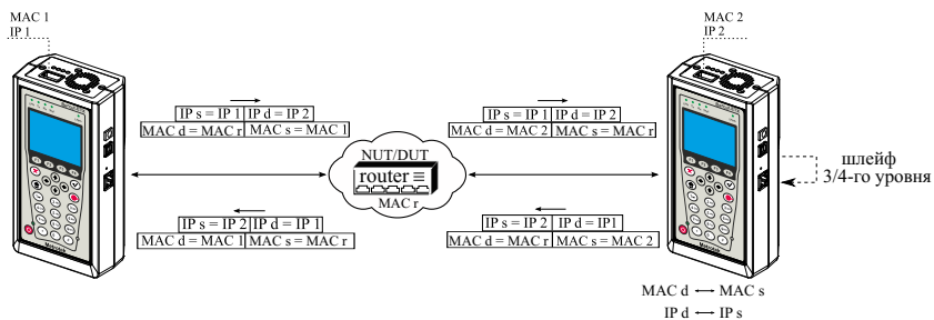
Рис. 6.2. Типовая схема подключения 2
