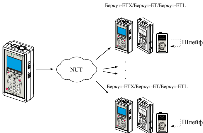
Рис. 11.1. Схема тестирования
