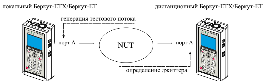
Рис. 14.6. Измерение джиттера. Схема 2
