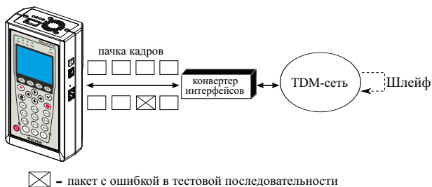
Рис. 13.12. Тестирование на канальном/сетевом уровне (вариант 3)
