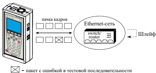
Рис. 13.11. Тестирование на канальном/сетевом уровне (вариант 2)
