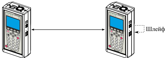
Рис. 13.9. Тестирование на физическом уровне (вариант 2)
