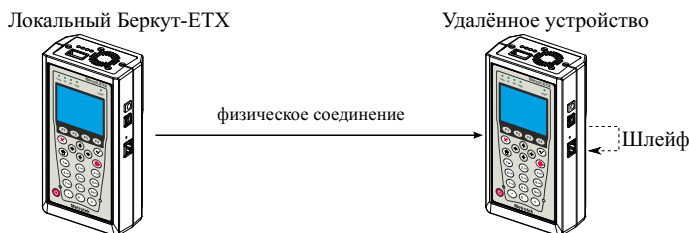
Рис. 10.1. Схема тестирования
