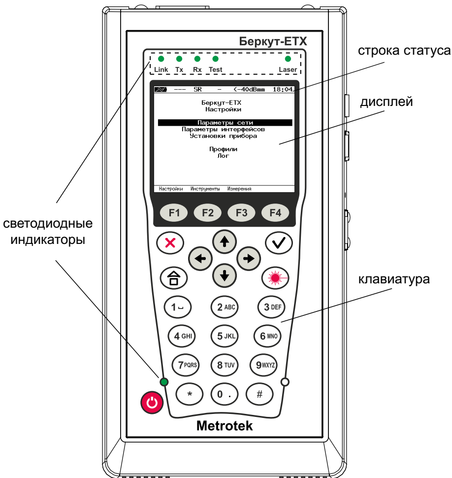
Рис. 4.1. Лицевая панель
