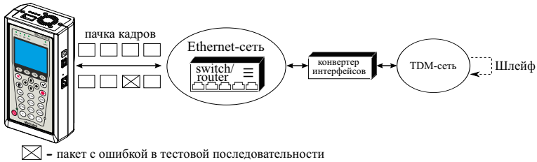
Рис. 13.10. Тестирование на канальном/сетевом уровне (вариант 1)
