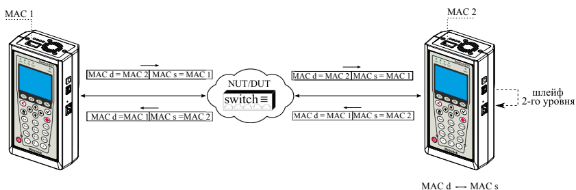
Рис. 6.1. Типовая схема подключения 1
