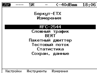
Рис. 5.6. Меню «Беркут-ЕТХ Измерения»
