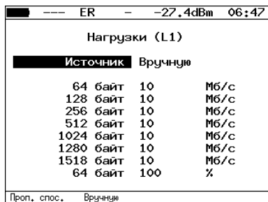
Рис. 7.10. Меню «Нагрузки (L1)»
