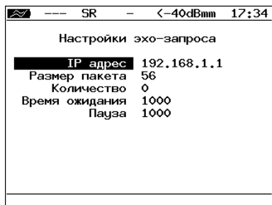
Рис. 13.3. Меню «Настройки эхо-запроса»
