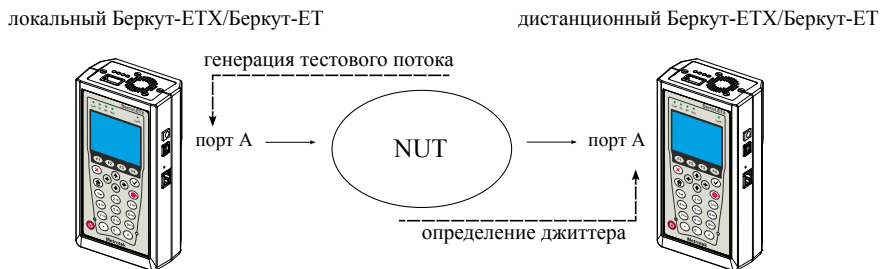
Рис. 15.6. Измерение джиттера. Схема 2
