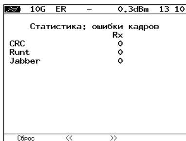
Рис. 16.5. Экран «Статистика: ошибки кадров»
