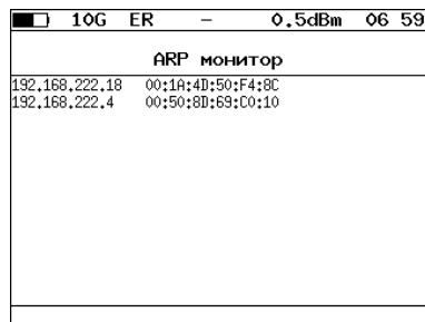
Рис. 13.11. Результаты тестирования
