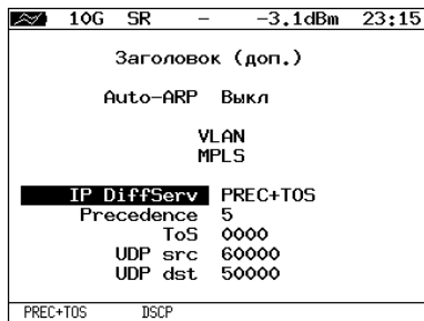
Рис. 7.4. Меню «Заголовок (доп.)»
