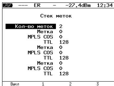
Рис. 19.4. Меню «Стек меток»
