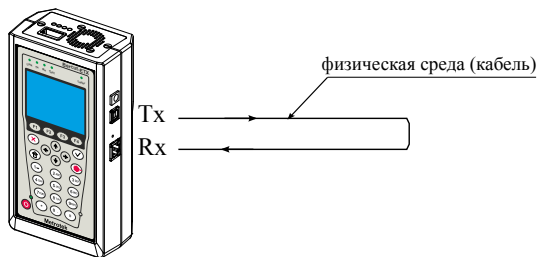
Рис. 14.8. Тестирование на физическом уровне (вариант 1)
