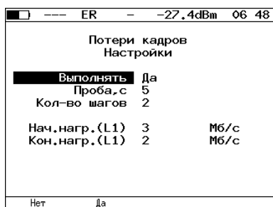
Рис. 7.11. Настройка параметров теста
