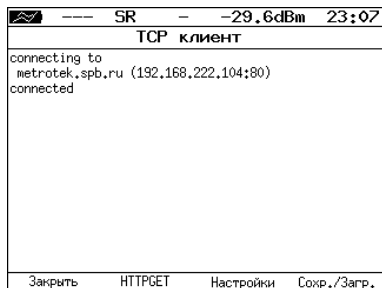
Рис. 13.14. Пример успешного соединения с узлом
