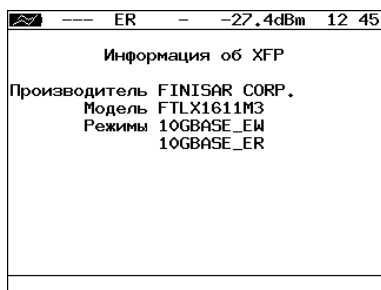
Рис. 20.4. Экран «Информация об XFP-модуле»
