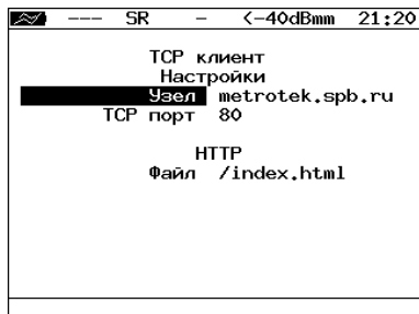
Рис. 13.13. Настройки теста «TCP клиент»
