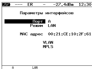
Рис. 19.1. Меню «Параметры интерфейсов»
