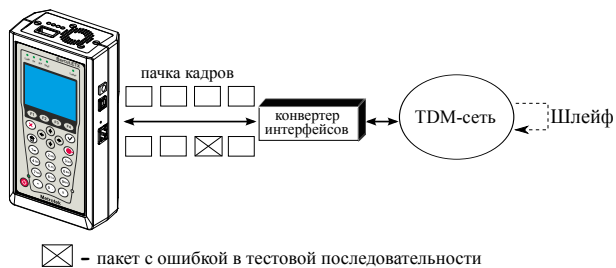
Рис. 14.12. Тестирование на канальном/сетевом уровне (вариант 3)
