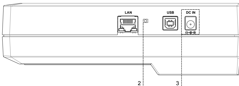
Рис. 5.3. Боковая панель тестера
