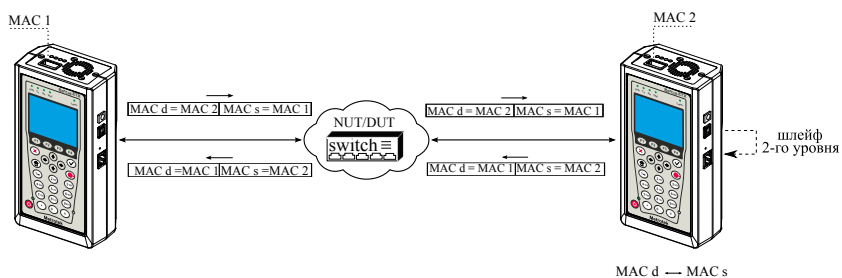
Рис. 7.1. Типовая схема подключения 1
