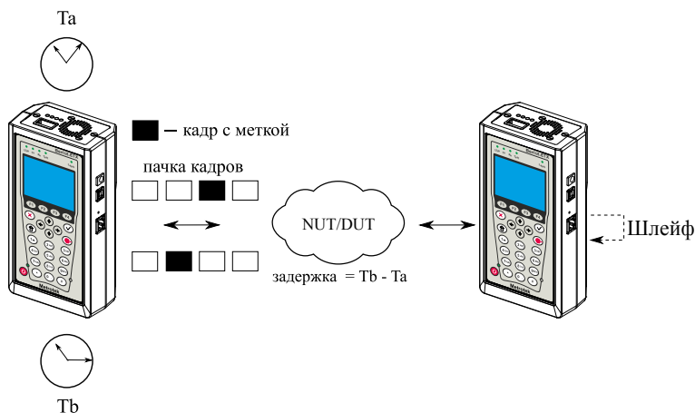
Рис. 6.2. Анализ задержки
