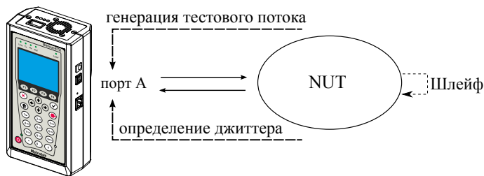
Рис. 15.5. Измерение джиттера. Схема 1
