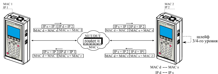
Рис. 7.2. Типовая схема подключения 2
