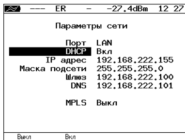
Рис. 18.1. Меню «Параметры сети»
