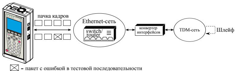
Рис. 14.10. Тестирование на канальном/сетевом уровне (вариант 1)
