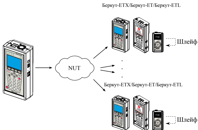
Рис. 12.1. Схема тестирования
