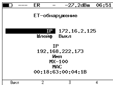
Рис. 12.3. Пример выполнения ET-обнаружения
