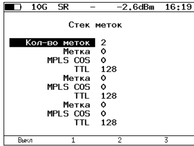
Рис. 9.10. Меню «Стек меток»
