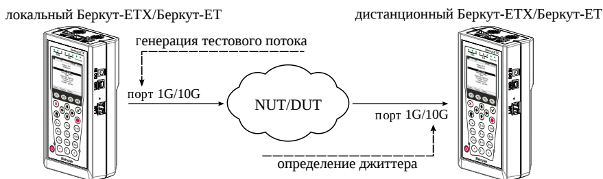
Рис. 19.3. Генерация постоянного трафика. Схема 2
