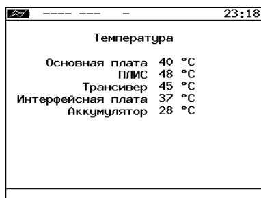
Рис. 24.5. Меню «Температура»
