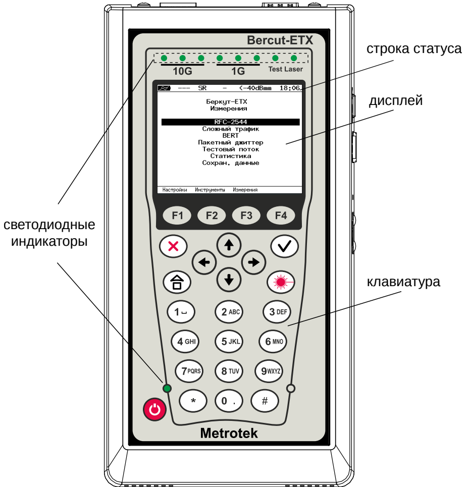
Рис. 5.1. Лицевая панель
