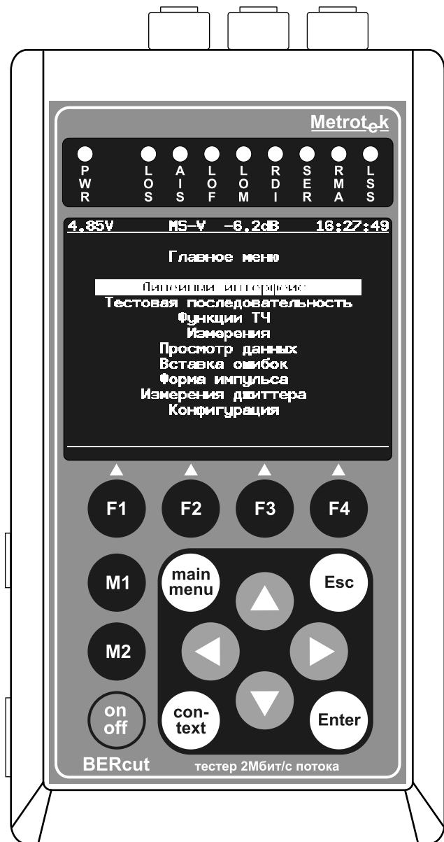
Внешний вид тестера Беркут–Е1
