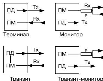
Рисунок 8.3. Режимы работы тестера
