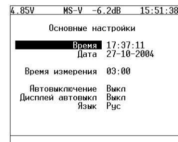
Рисунок 8.19. Меню «Основные настройки»
