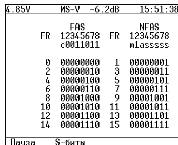
Рисунок 8.14. Меню «FAS/NFAS»
