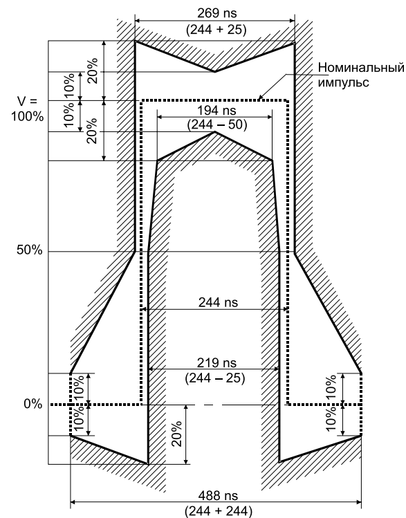
Рисунок 8.21. Шаблон импульса G.703 (2048 кбит/с)
