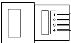
Рисунок 4.4. Схема контактов разъема гарнитуры
