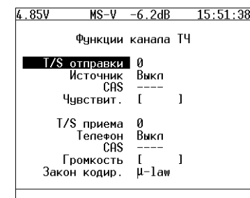
Рисунок 8.6. Меню «Функции канала ТЧ»
