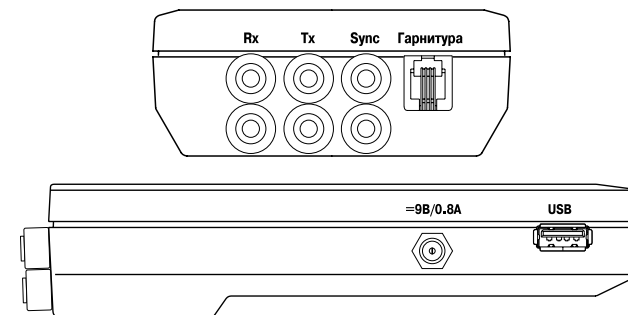
Рисунок 4.2. Вид корпуса тестера
