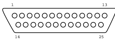
Рис. А.2. Схематическое изображение интерфейса адаптера В4-ДА-А2 (вилка)
