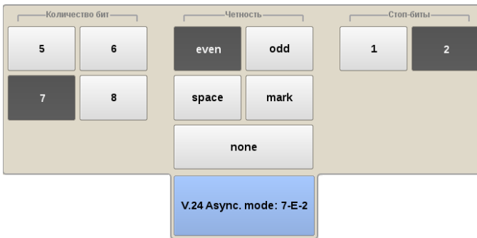
Рис. 5.3. Окно «V.24 Async. mode»
