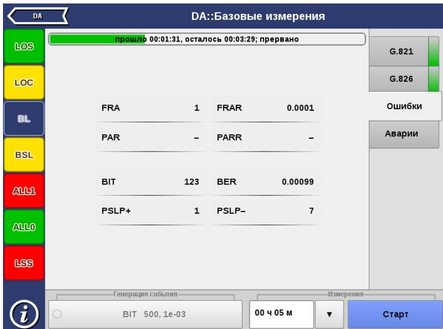
Рис. 6.8. Вкладка «Ошибки»
