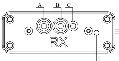
Рис. А.5. Интерфейс адаптера С1-И (приемная часть)
