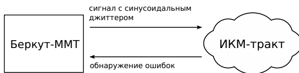
Рис. 9.3. Измерение максимально допустимого джиттера
