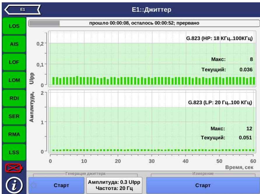
Рис. 9.5. Результаты измерения джиттера
