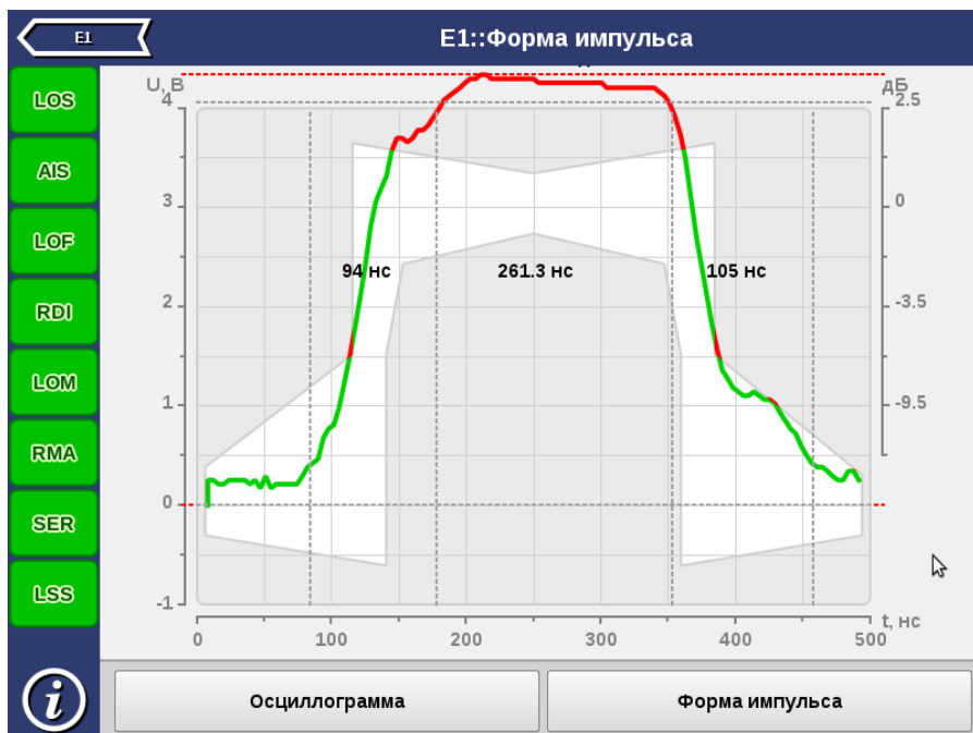
Рис. 10.1. Приложение «E1 – Форма импульса»
