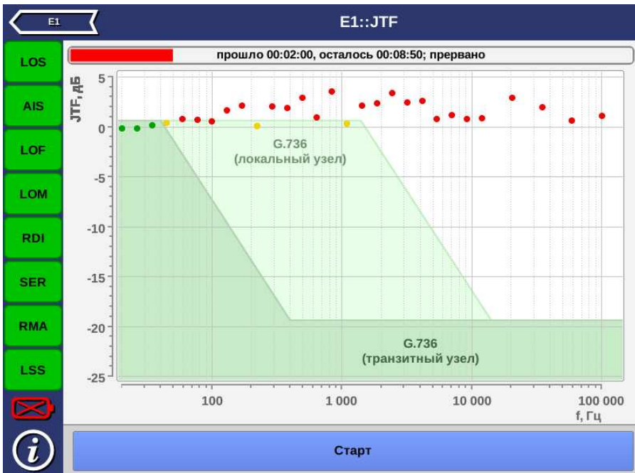
Рис. 9.6. Результаты измерения JTF
