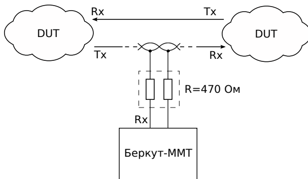
Рис. 5.5. Использование защитных резисторов
