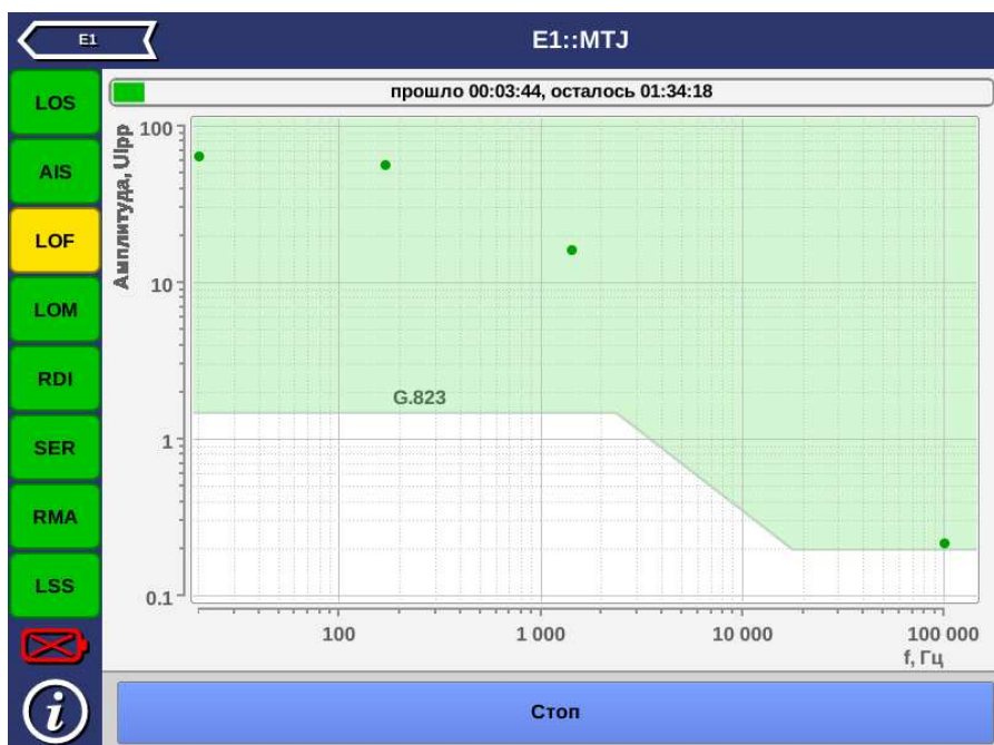
Рис. 9.7. Результаты измерения МТЖ
