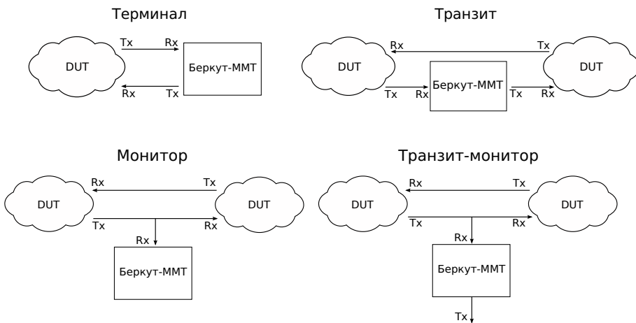
Рис. 5.2. Режимы работы прибора
