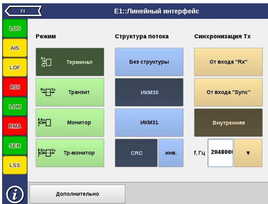
Рис. 5.1. Приложение «Е1 — Линейный интерфейс»
