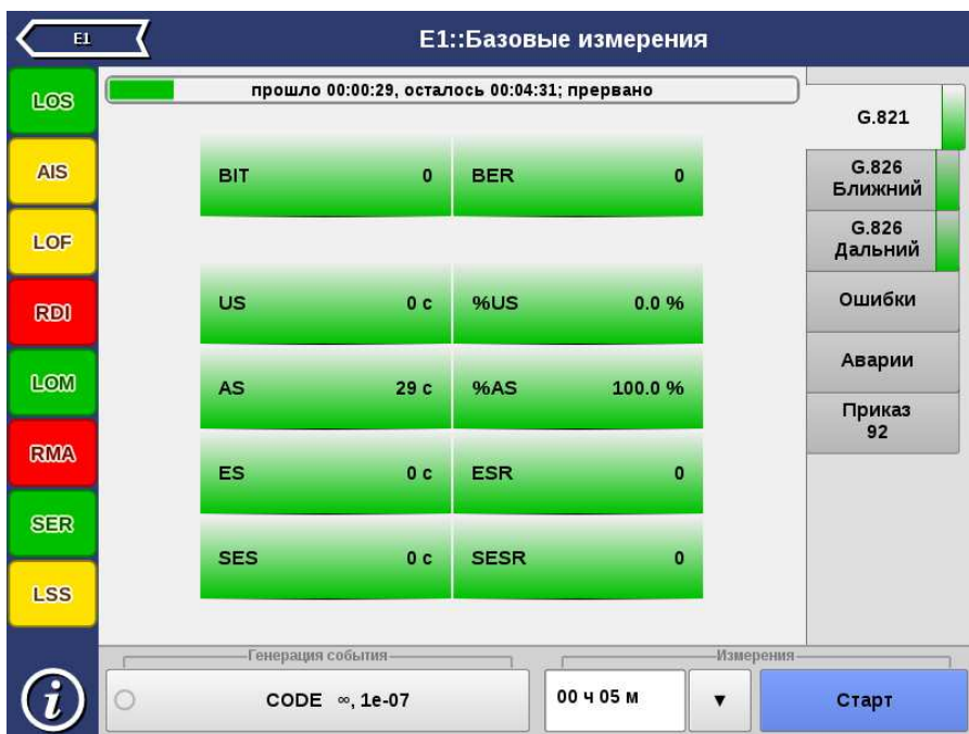
Рис. 7.7. Результаты измерений G.821
