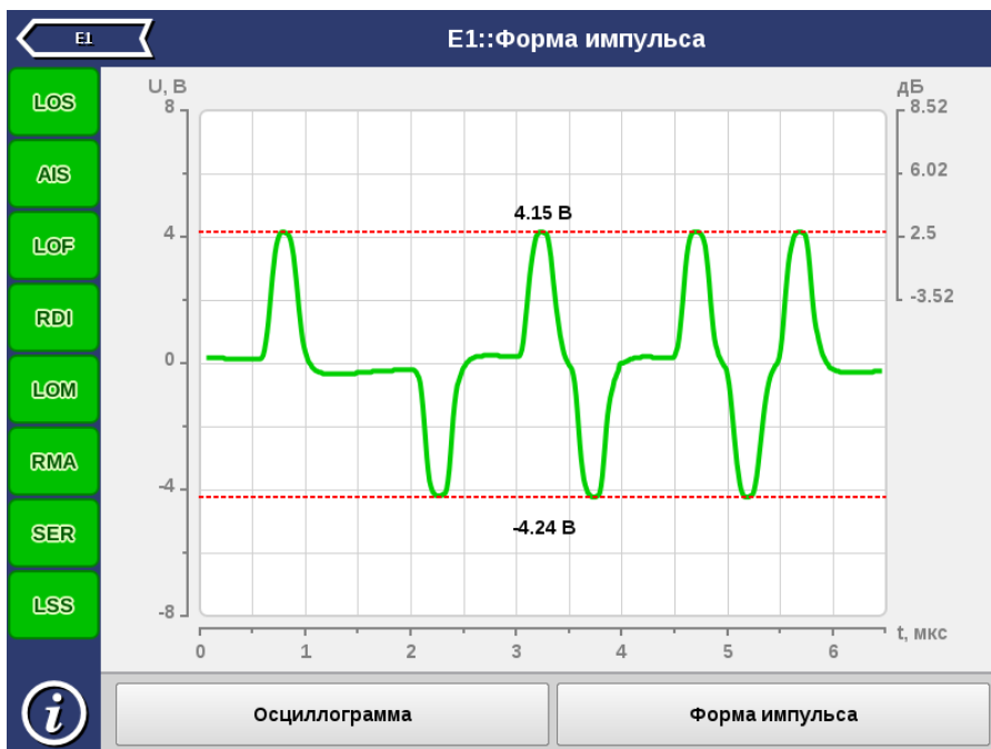
Рис. 10.2. Отображение осциллограммы
