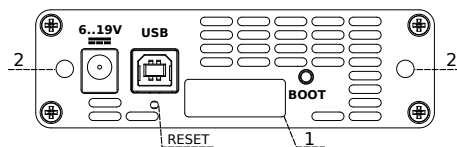
Рис. 3.2. Задняя панель модуля E1
