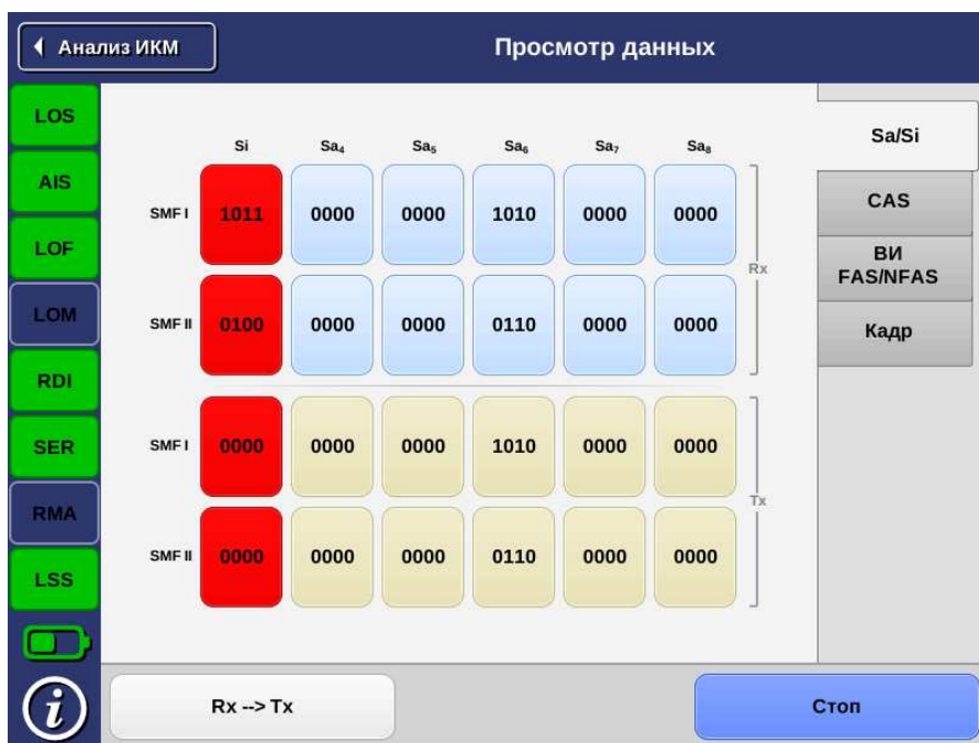
Рис. 13.1. Вкладка Sa/Si
