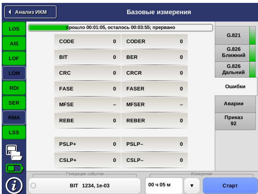
Рис. 8.10. Вкладка «Ошибки»
