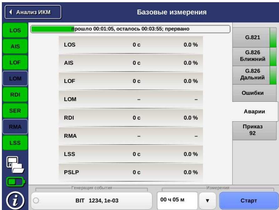
Рис. 8.11. Вкладка «Аварии»
