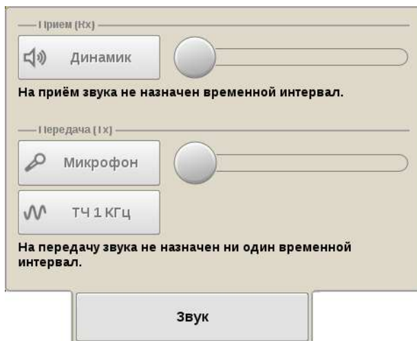
Рис. 7.4. Окно «Звук»
