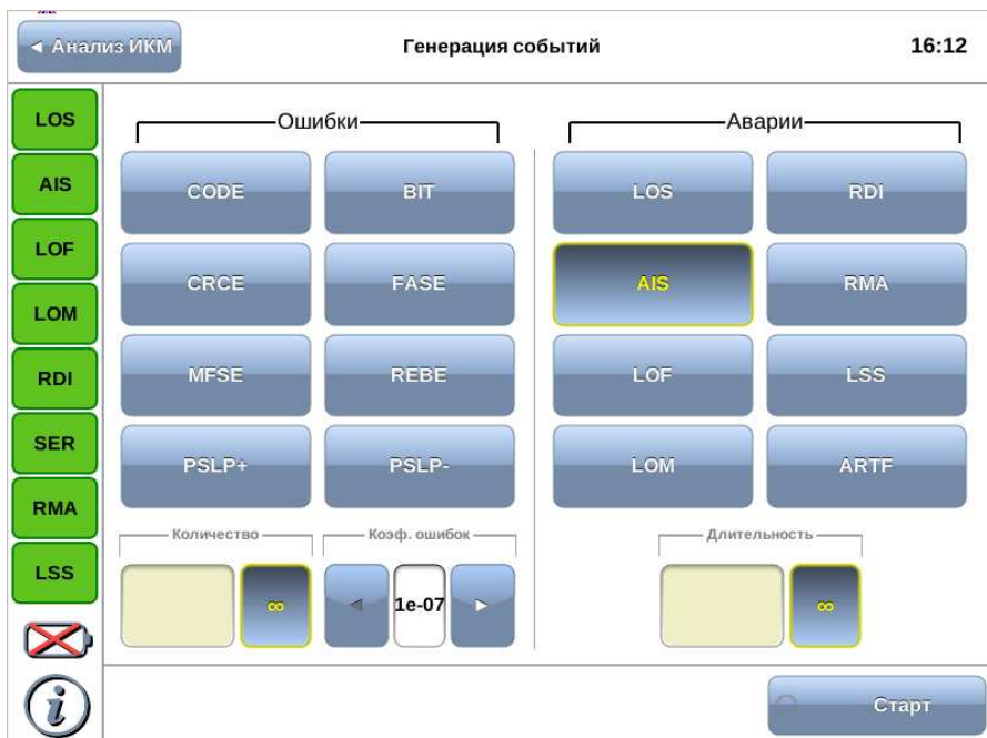
Рис. 10.1. Приложение «Е1 — Генерация событий»
