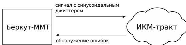
Рис. 11.3. Измерение максимально допустимого джиттера
