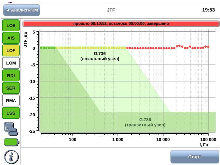
Рис. 11.6. Результаты измерения JTF
