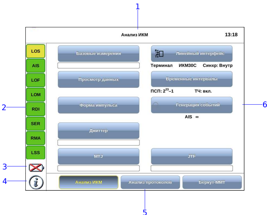
Рис. 5.1. Главное меню
