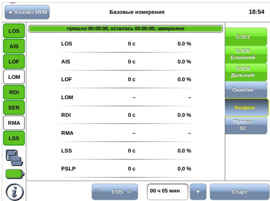
Рис. 8.11. Вкладка «Аварии»
