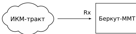
Рис. 11.1. Измерение джиттера на выходе сетевого элемента
