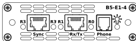
Рис. 4.1. Передняя панель модуля E1
