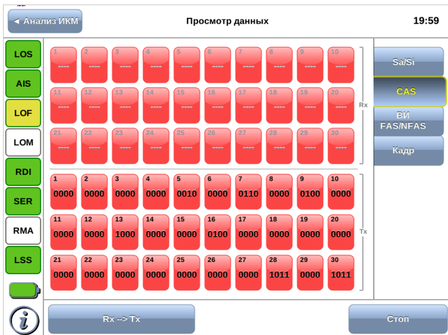
Рис. 13.2. Вкладка «Сигнальные биты CAS»
