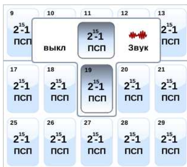
Рис. 7.2. Диалоговое окно
