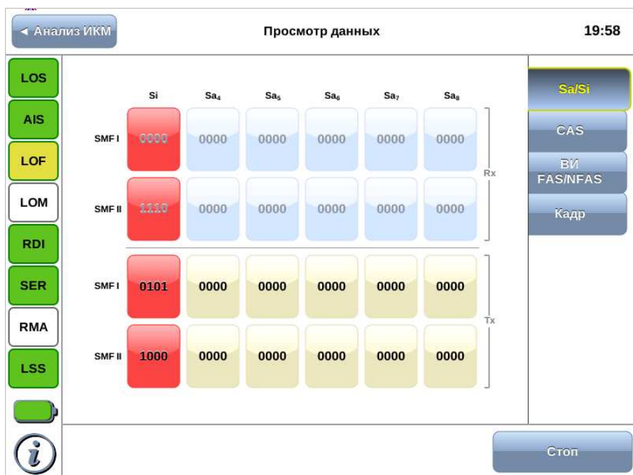
Рис. 13.1. Вкладка Sa/Si
