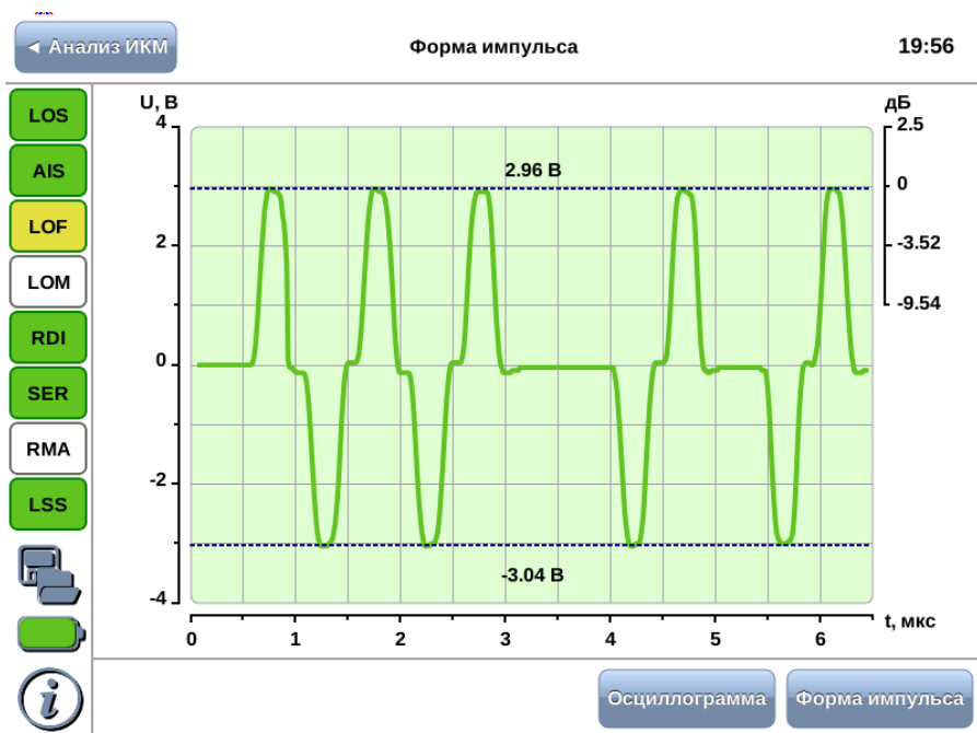
Рис. 12.2. Отображение осциллограммы
