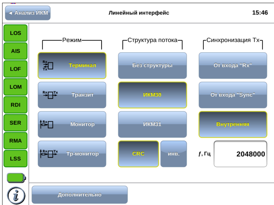
Рис. 6.1. Приложение «E1 — Линейный интерфейс»
