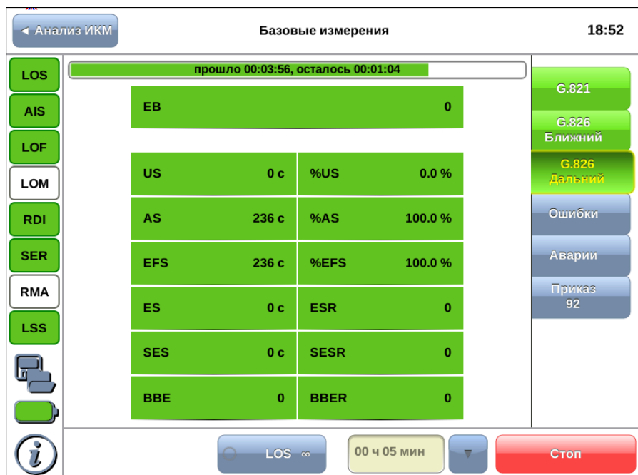
Рис. 8.9. Результаты измерений G.826 (дальний конец)
