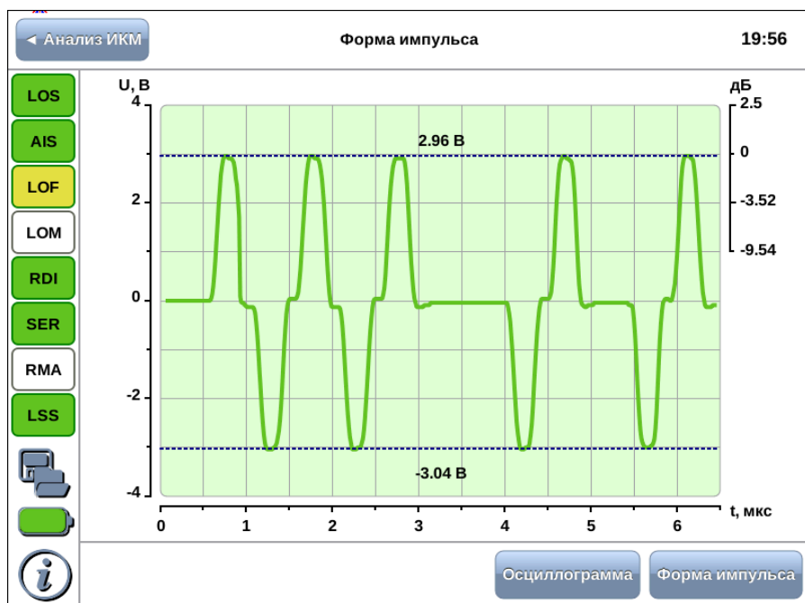
Рис. 11.2. Отображение осциллограммы
