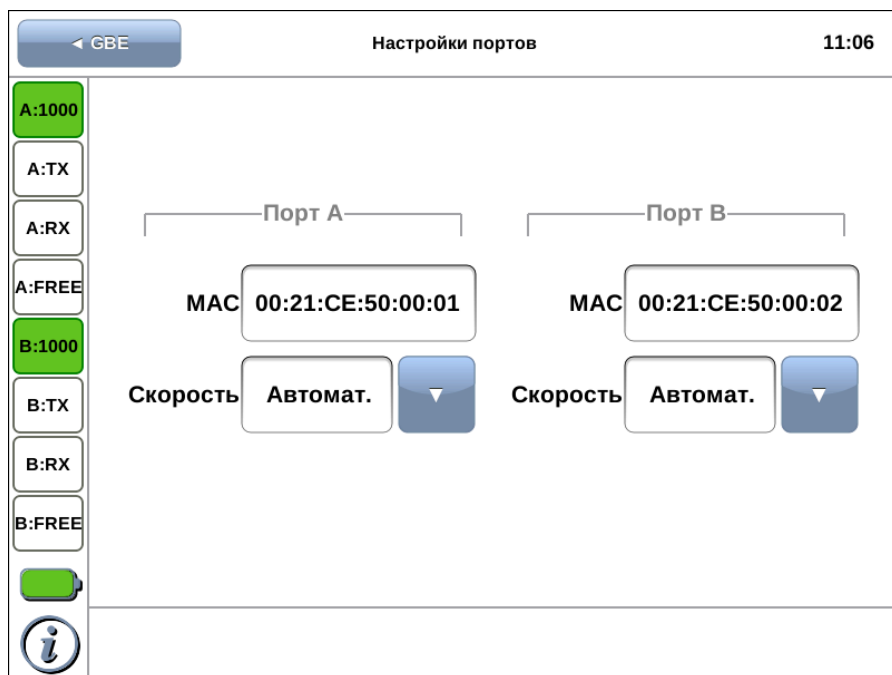
Рис. 17.1. Режим «Настройки портов»
