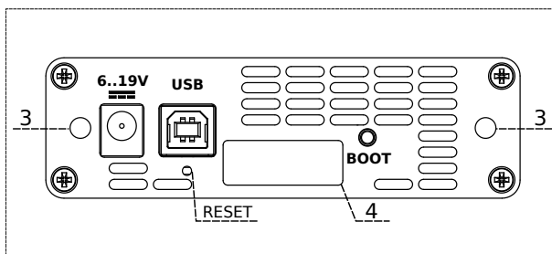
Рис. 5.2. Задняя панель модуля B5-GBE
