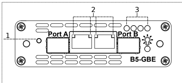
Рис. 5.1. Передняя панель модуля B5-GBE
