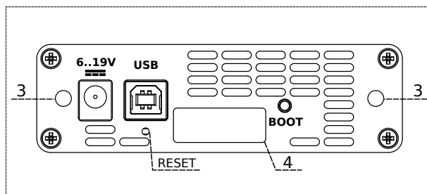
Рис. 5.2. Задняя панель модуля B5-GBE
