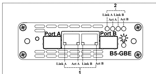
Рис. 5.1. Передняя панель модуля B5-GBE (первая модификация)
