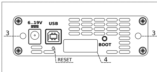
Рис. 5.3. Задняя панель модуля В5-GBE
