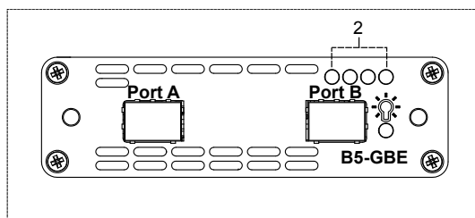
Рис. 5.2. Передняя панель модуля B5-GBE (вторая модификация)
