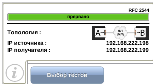
Рис. 7.2. Статусная панель
