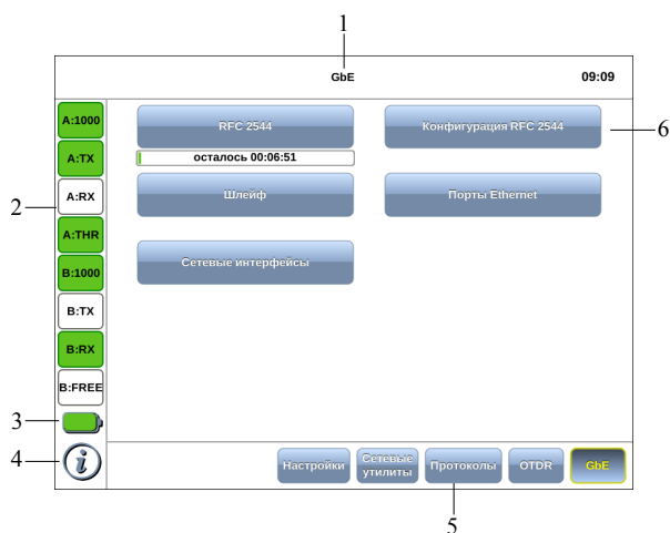
Рис. 7.1. Главное меню
