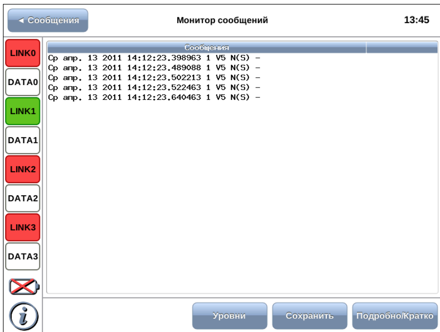
Рис. 7.5. Окно расшифровки
