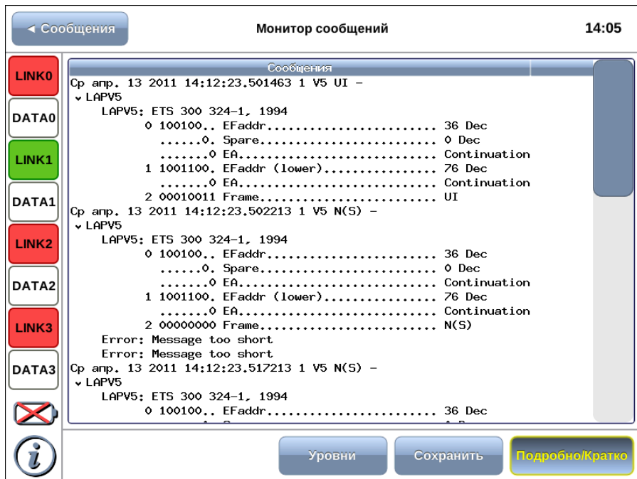
Рис. 8.4. Окно просмотра
