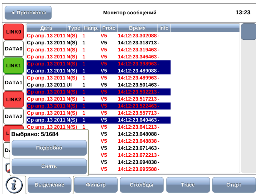
Рис. 7.4. Выделение сообщений
