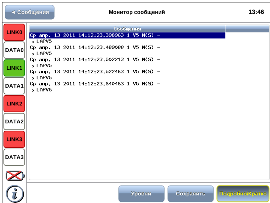
Рис. 7.6. Декодированные сообщения
