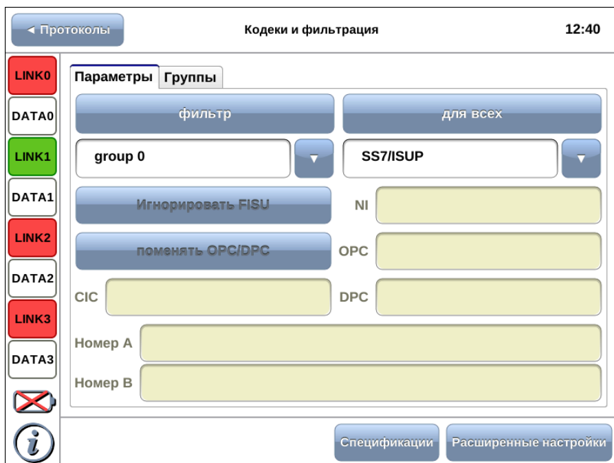
Рис. 5.2. Вкладка Параметры
