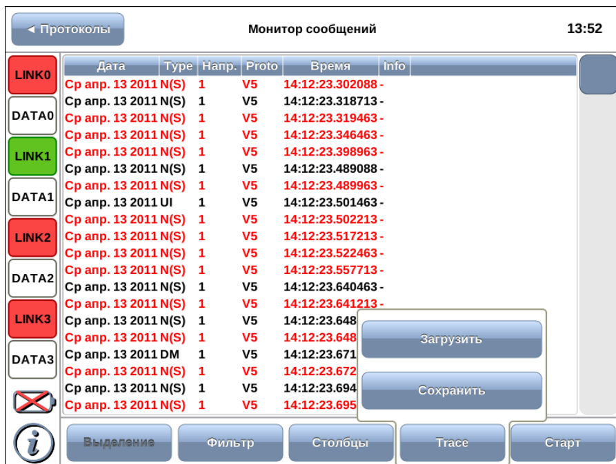
Рис. 8.1. Сохранение/загрузка трейс-файлов
