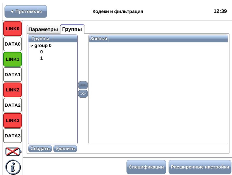
Рис. 5.1. Вкладка Группы
