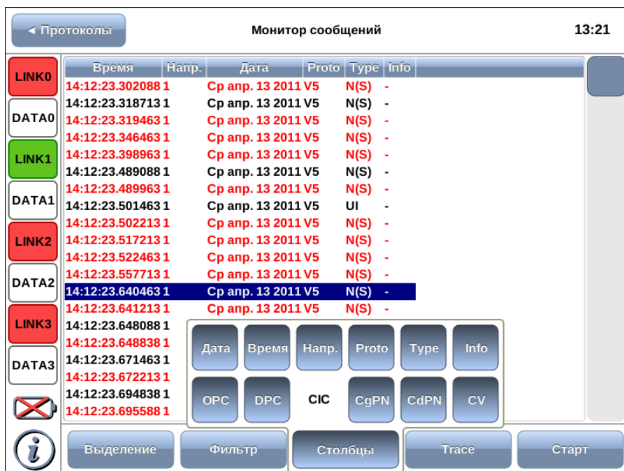
Рис. 7.3. Окно «Столбцы»
