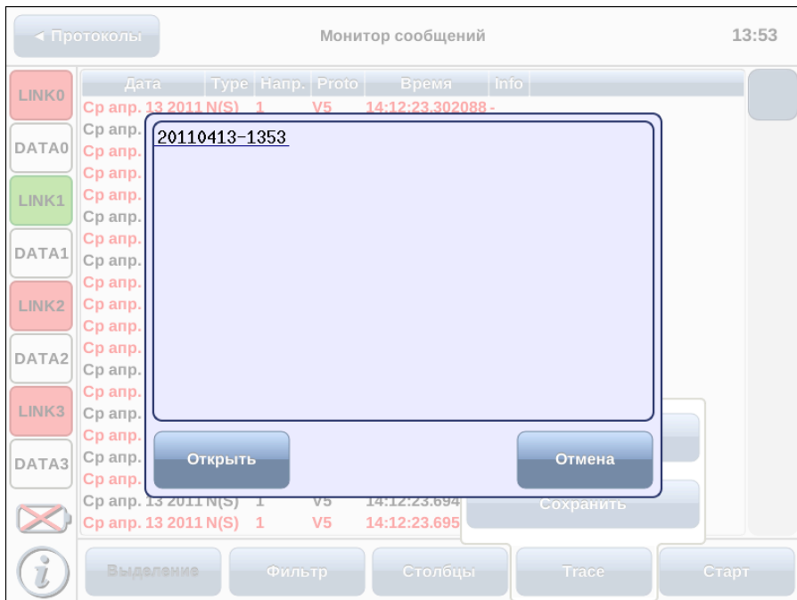
Рис. 8.2. Выбор трейс-файла
