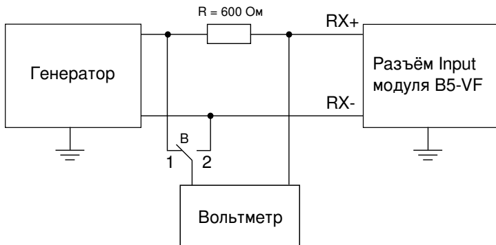
Рис. 9.6. Схема подключения
