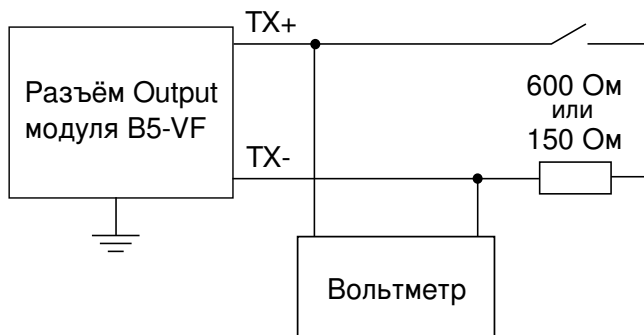
Рис. 10.3. Схема подключения
