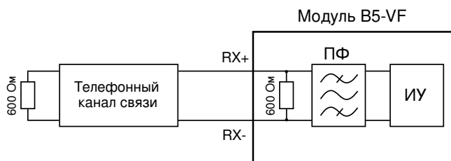
Рис. 9.1. Схема измерения уровня псофометрического шума
