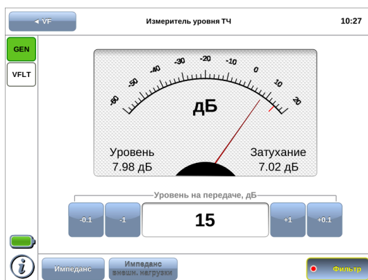
Рис. 8.5. Включение фильтра
