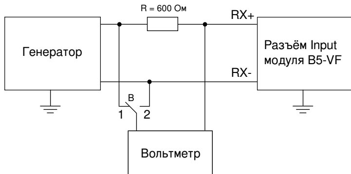
Рис. 10.6. Схема подключения
