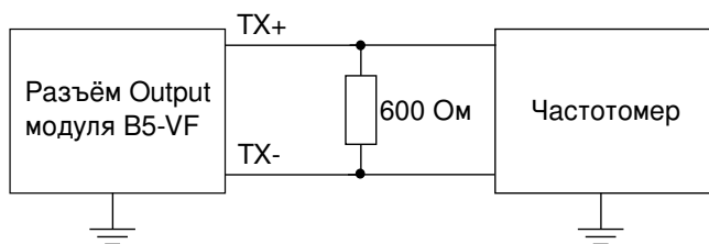
Рис. 10.1. Схема подключения
