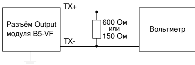
Рис. 10.2. Схема подключения
