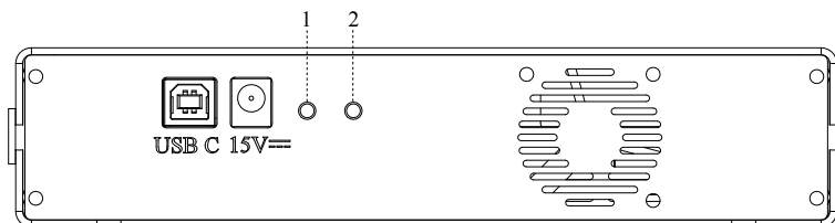
Рис. 4.2. Задняя панель прибора Беркут-МХ
