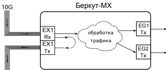
Рис. 7.3. Типовая схема подключения 3
