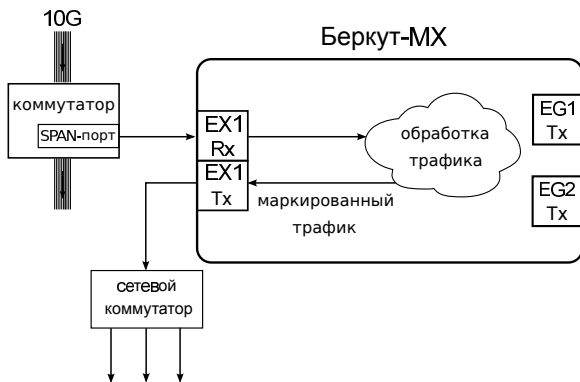
Рис. 7.5. Типовая схема подключения 5
