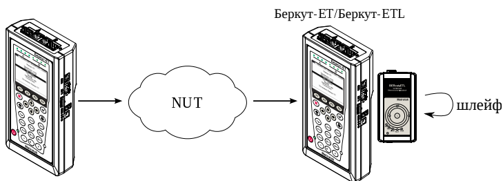
Рис. 9.1. Схема тестирования
