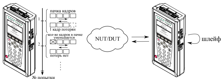
Рис. 4.4. Анализ предельной нагрузки
