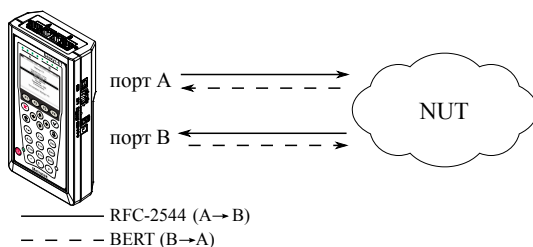
Рис. 3.1. Схема подключения
