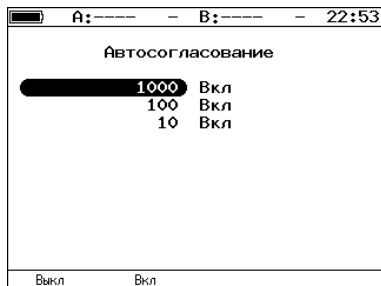
Рис. 24.2. Меню «Автосогласование»
