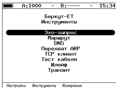
Рис. 2.2. Меню «Беркут-ЕТ Инструменты»
