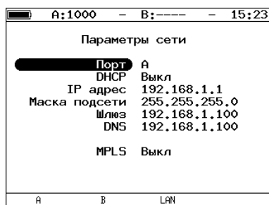
Рис. 23.1. Меню «Параметры сети»
