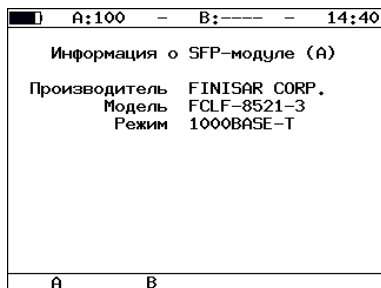
Рис. 25.5. Экран «Информация о SFP-модуле»
