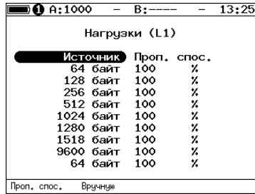
Рис. 7.3. Меню «Нагрузки (L1)»
