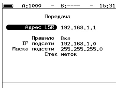
Рис. 24.4. Меню «Передача»
