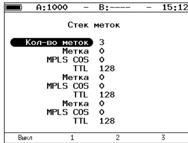
Рис. 20.2. Меню «Стек меток»
