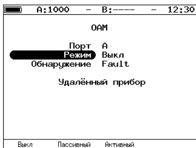
Рис. 12.1. Меню «OAM»
