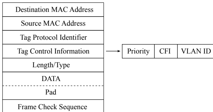
Рис. А.2. Структура Ethernet-кадра, содержащего VLAN-метку
