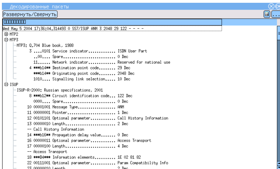
Рис. 5.11. Настройка уровня детализации
