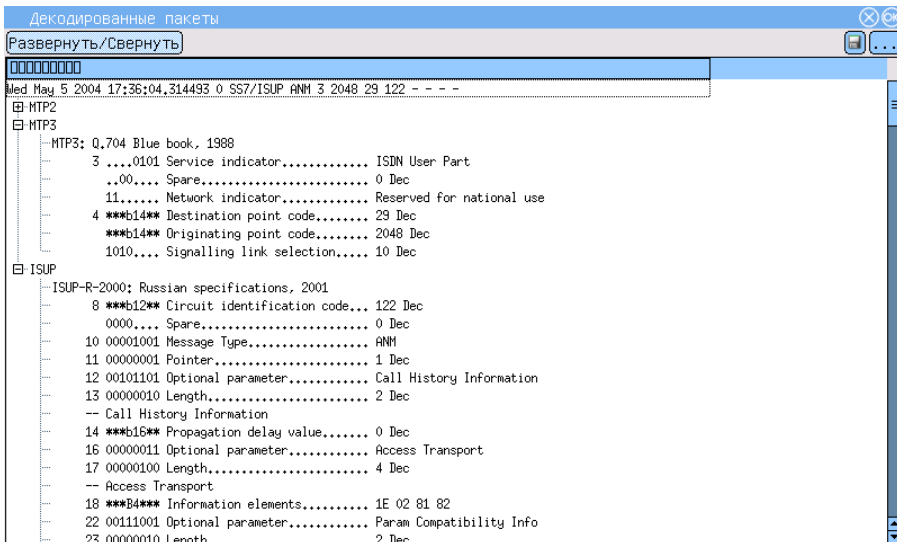
Рис. 5.10. Декодирование данных: подробная расшифровка
