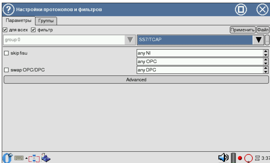
Рис. 6.7. Подсистема фильтров: настройка по протоколам SS7/ТСАР
