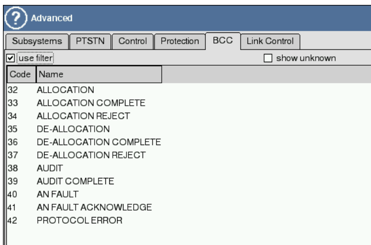
Рис. 6.15. Фильтрация по сообщениям протокола BCC
