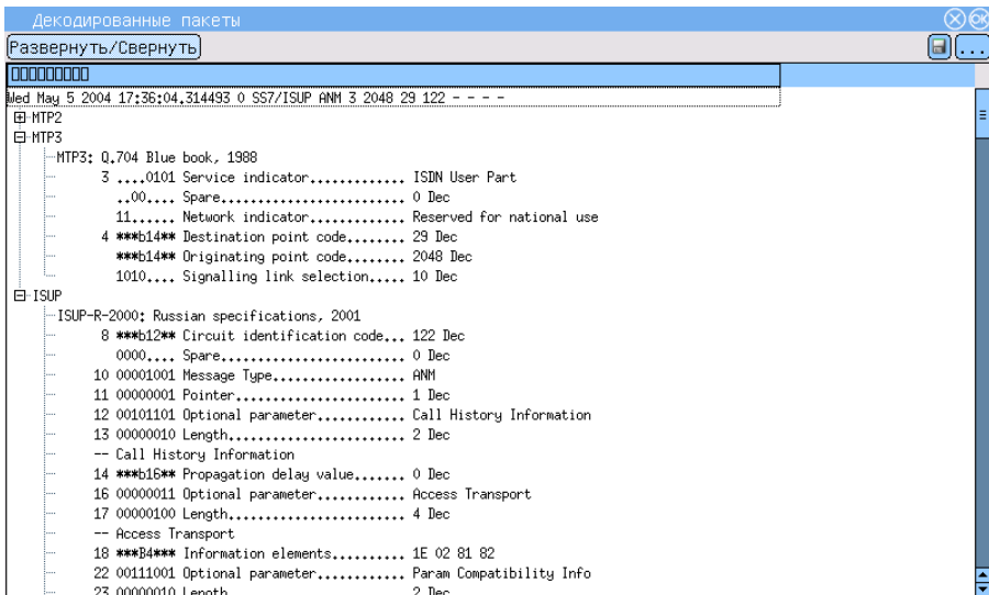
Рис. 5.13. Декодированные пакеты: развёрнутый вид сообщений
