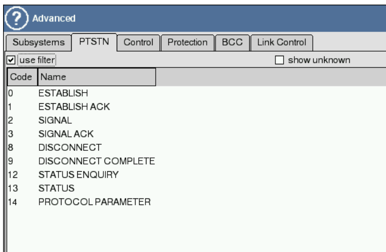
Рис. 6.12. Фильтрация по сообщениям протокола PTSTN
