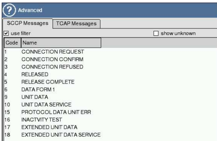
Рис. 6.9. Фильтрация сообщений по типу SCCP
