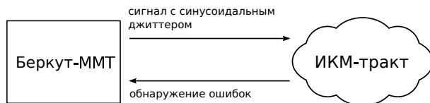
Рис. 10.3. Измерение максимально допустимого джиттера
