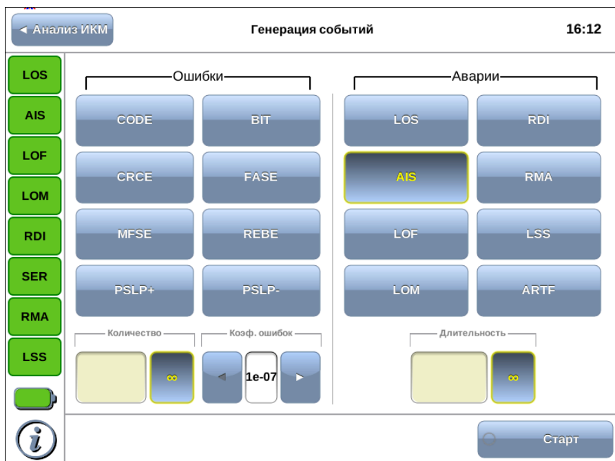
Рис. 9.1. Приложение «E1 — Генерация событий»
