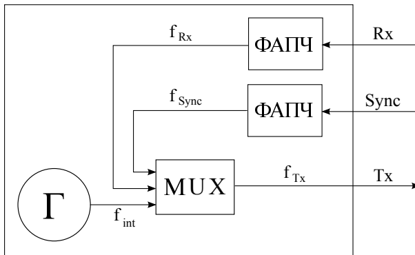
Рис. 6.3. Схема мультиплексирования частоты передачи
