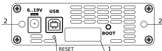
Рис. 4.2. Задняя панель модуля E1
