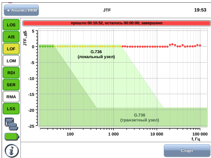
Рис. 10.6. Результаты измерения JTF
