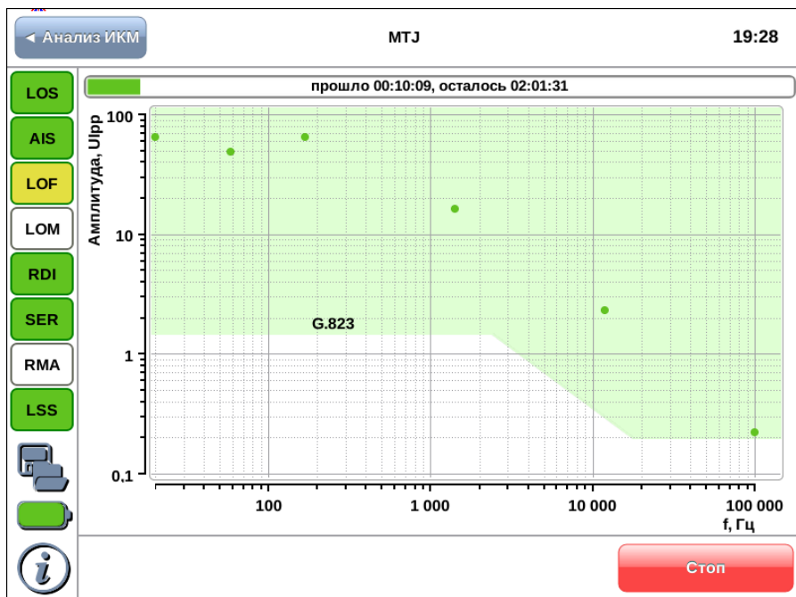
Рис. 10.7. Результаты измерения МТJ
