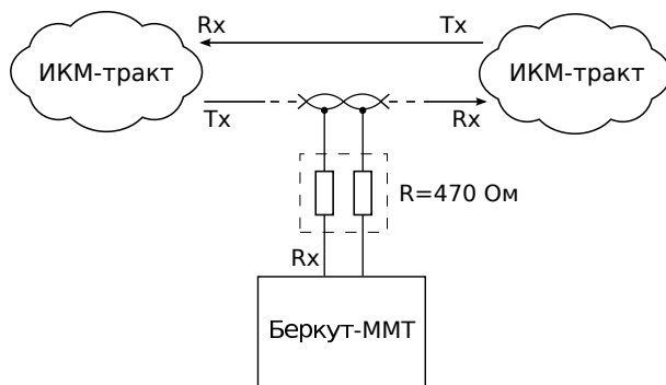
Рис. 6.6. Использование защитных резисторов
