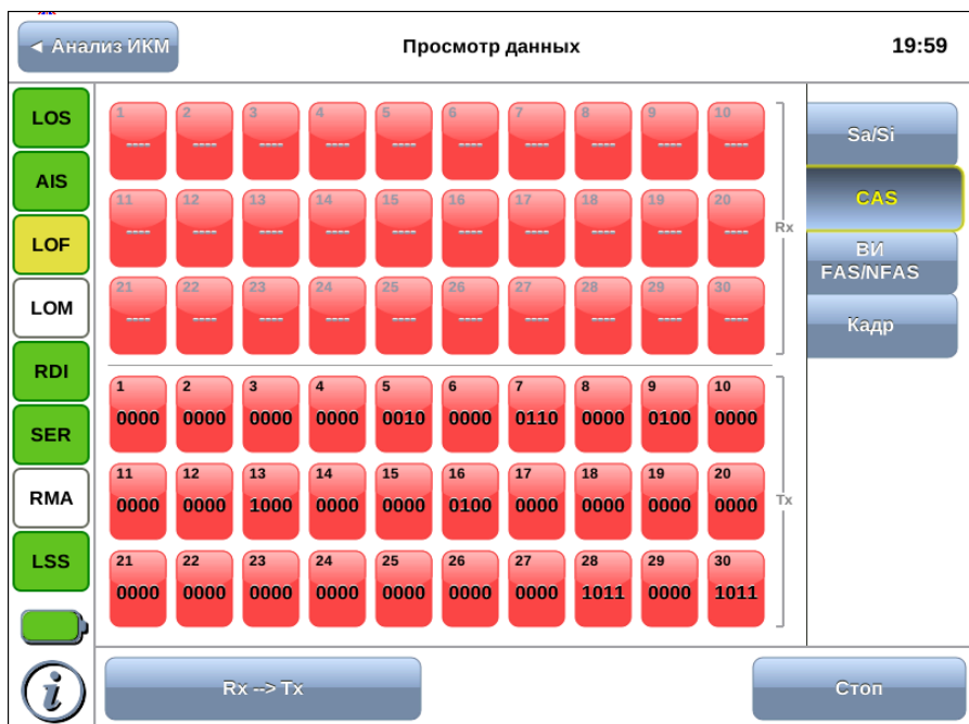
Рис. 12.2. Вкладка «Сигнальные биты CAS»
