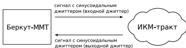
Рис. 10.2. Измерение передаточной характеристики джиттера
