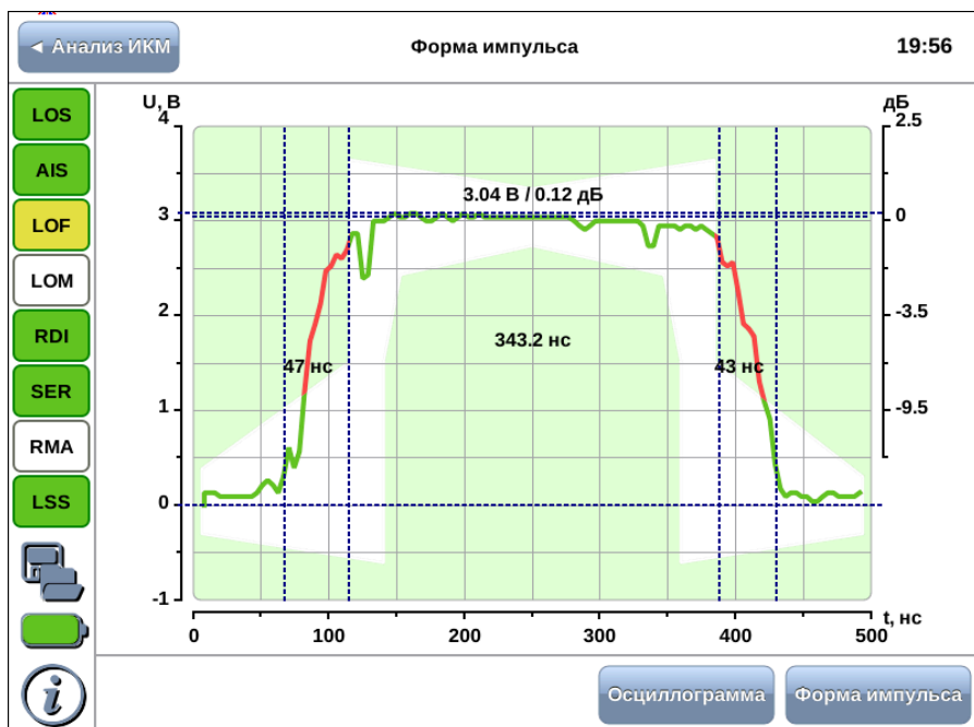
Рис. 11.1. Приложение «E1 – Форма импульса»
