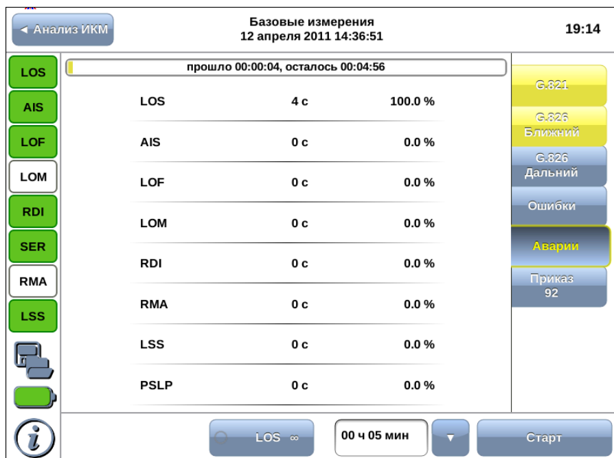
Рис. 13.3. Отчёт о проведённых измерениях
