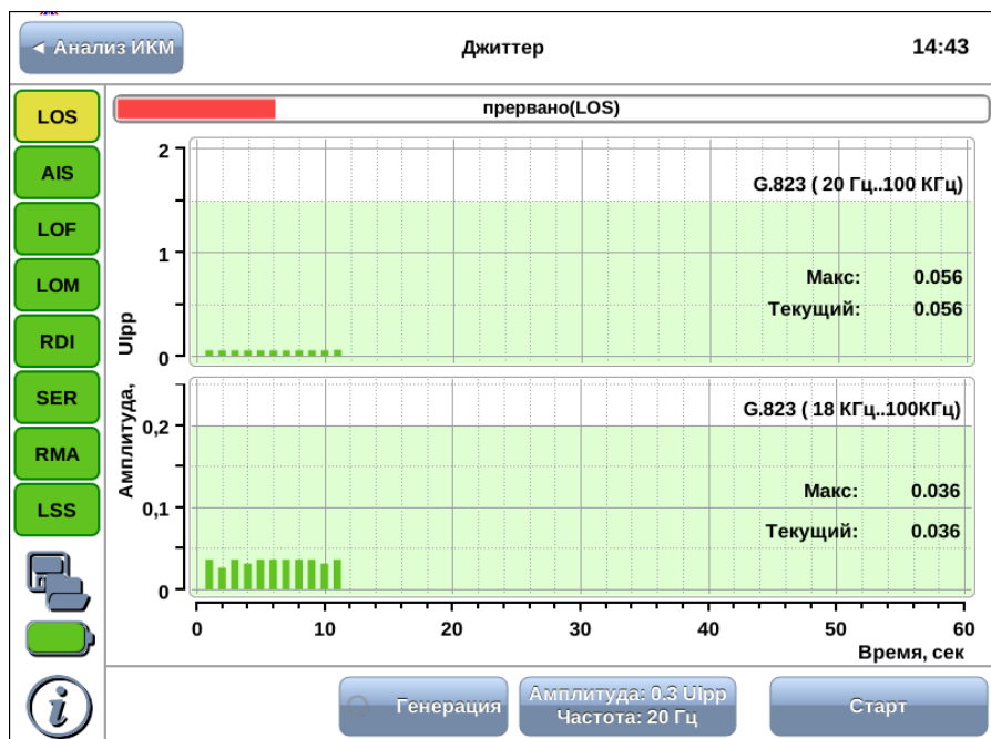
Рис. 10.5. Результаты измерения джиттера
