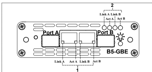
Рис. 5.1. Передняя панель модуля B5-GBE (первая модификация)
