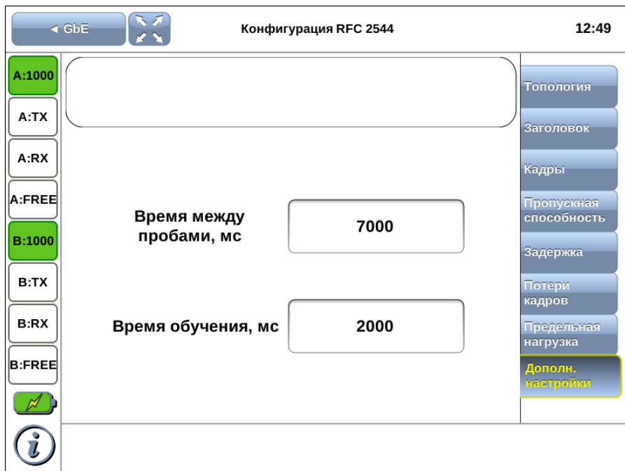
Рис. 12.5. Вкладка «Дополнительные настройки»
