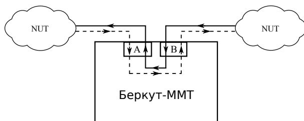
Рис. 17.1. Подключение в режиме «Транзит»
