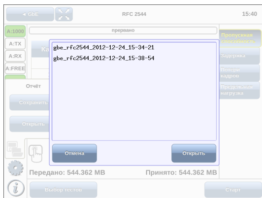
Рис. 20.2. Список сохранённых отчётов
