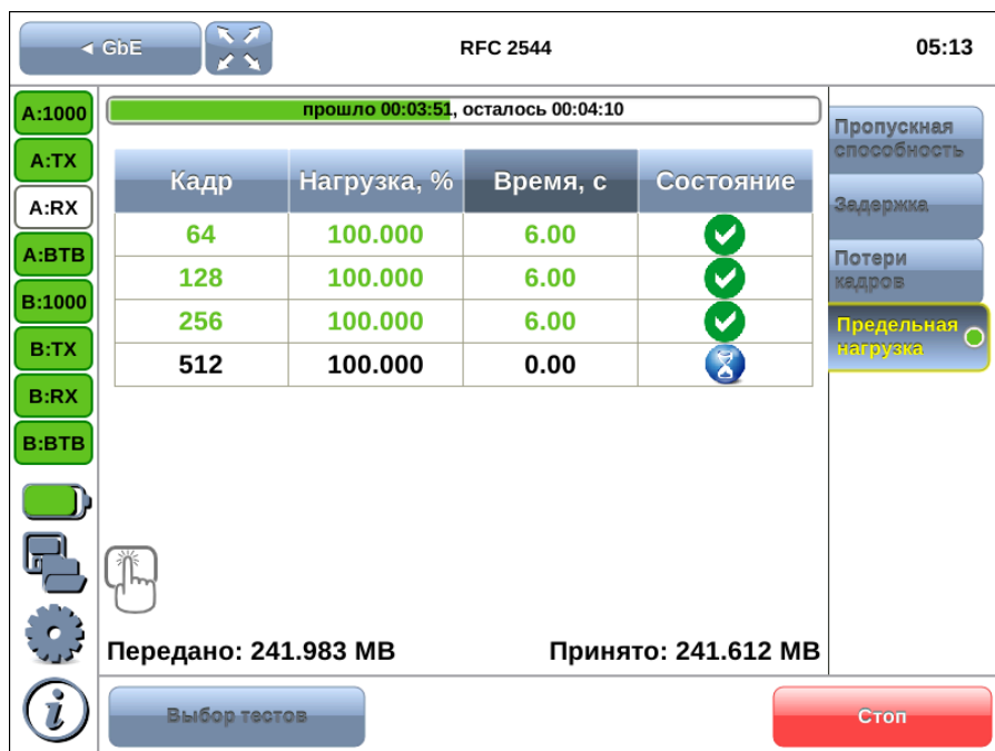
Рис. 14.7. Результаты теста: таблица
