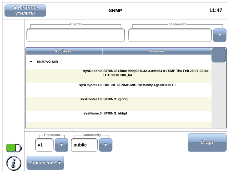
Рис. 18.1. SNMP: пример результатов тестирования
