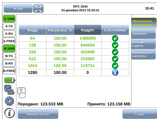
Рис. 20.3. Отчёт о проведённых измерениях
