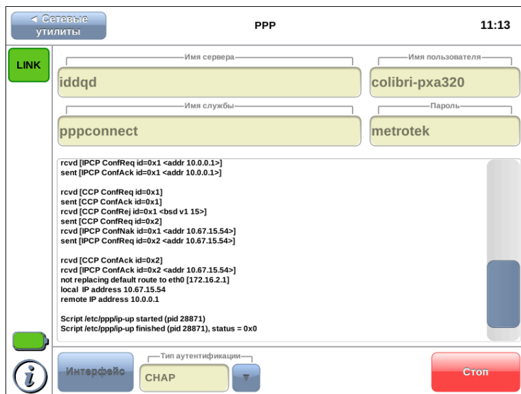
Рис. 18.2. PPP: пример результатов тестирования
