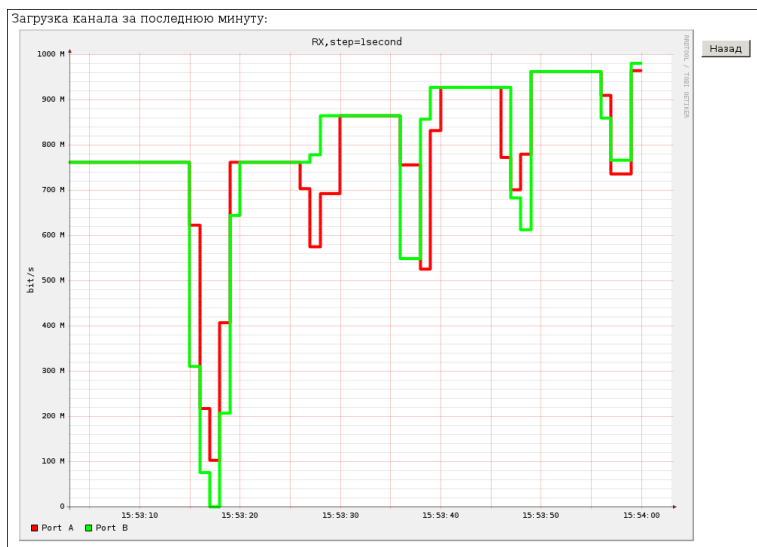
Рис. 17.2. График загрузки канала
