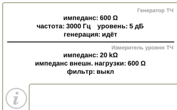
Рис. 6.2. Статусная панель
