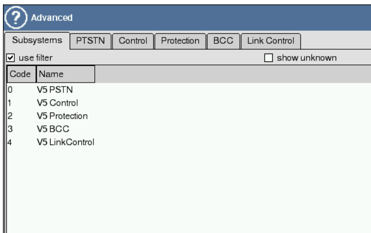
Рис. 5.22. Фильтрация по подсистемам V5
