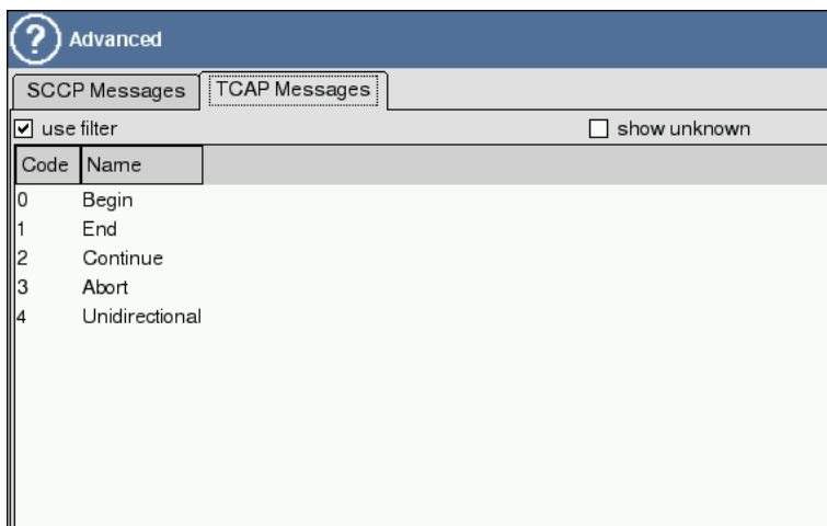
Рис. 5.21. Дополнительные настройки SS7/TCAP: TCAP
