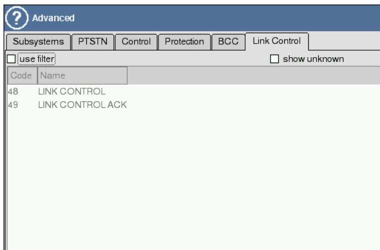
Рис. 5.27. Дополнительная настройка фильтров для V5: Link Control
