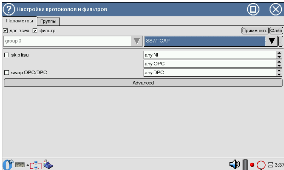
Рис. 5.16. Подсистема фильтров: настройка по протоколам SS7/TCAP
