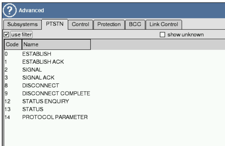
Рис. 5.23. Дополнительная настройка фильтров для V5: PTSTN
