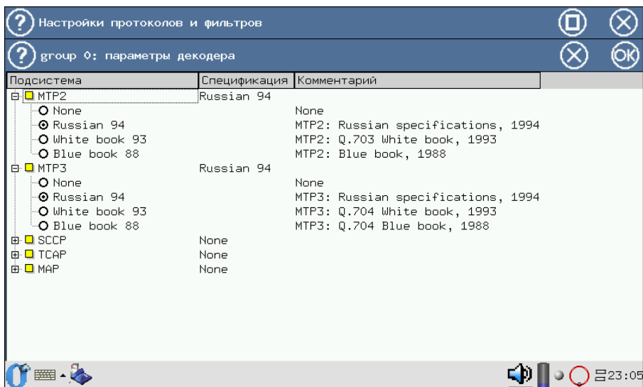
Рис. 5.17. Меню выбора декодера для протокола SS7/TCP
