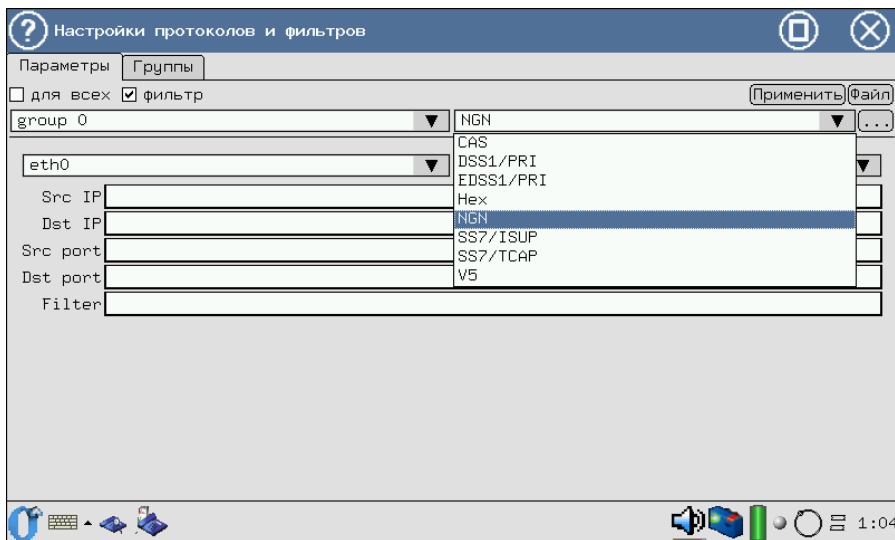
Рис. 5.10. Подсистема фильтров: настройка декодера NGN
