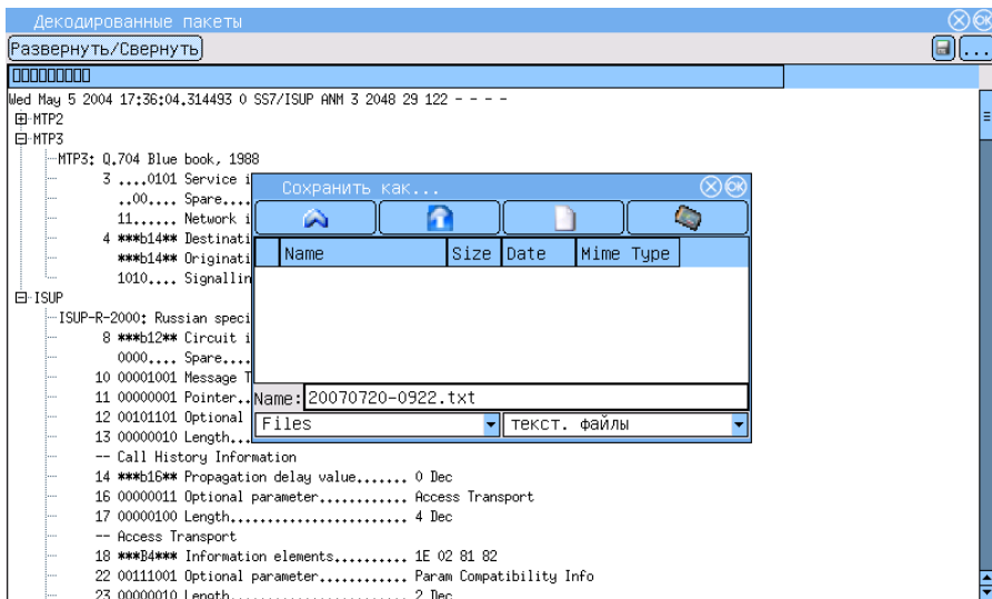
Рис. 6.18. Декодирование данных: запись в файл
