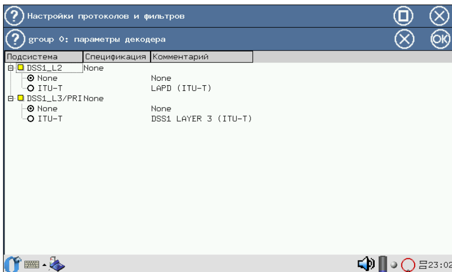
Рис. 5.6. Меню выбора декодера для протокола DSS1/PRI
