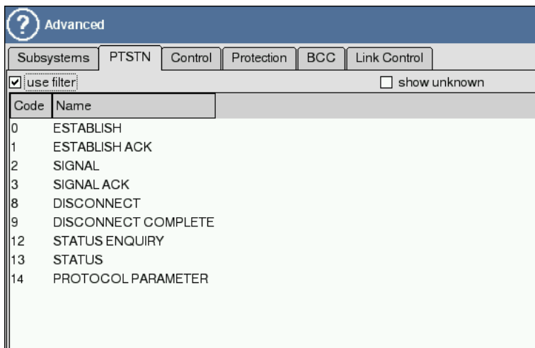
Рис. 5.23. Дополнительная настройка фильтров для V5: PSTN
