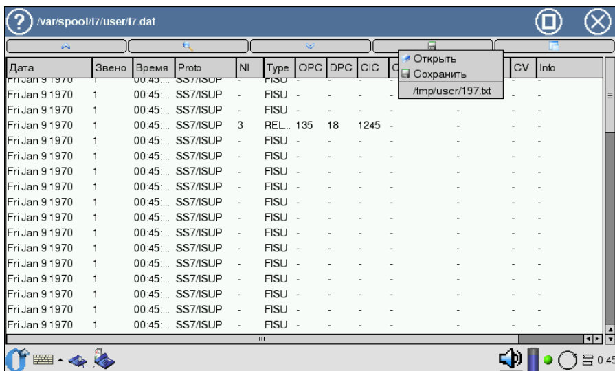
Рис. 6.19. Сохранение данных
