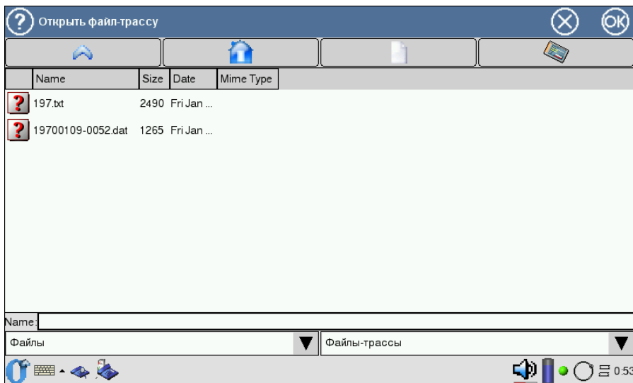
Рис. 6.21. Открытие файл-трассы
