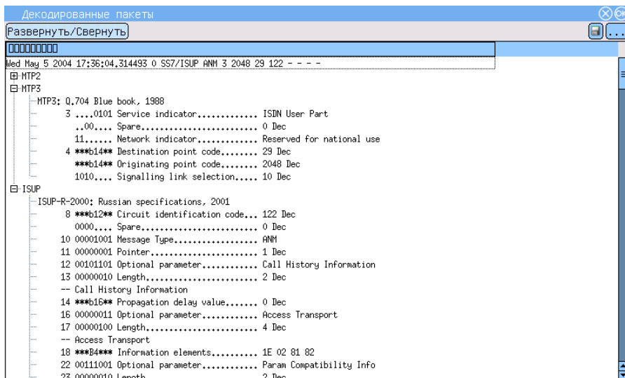
Рис. 6.14. Декодирование данных: подробная расшифровка
