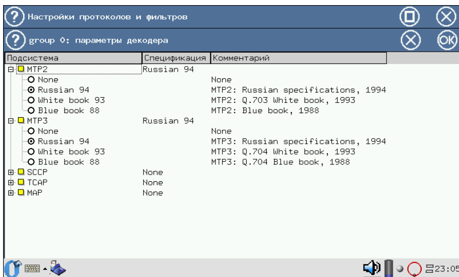
Рис. 5.17. Меню выбора декодера для протокола SS7/TCAP
