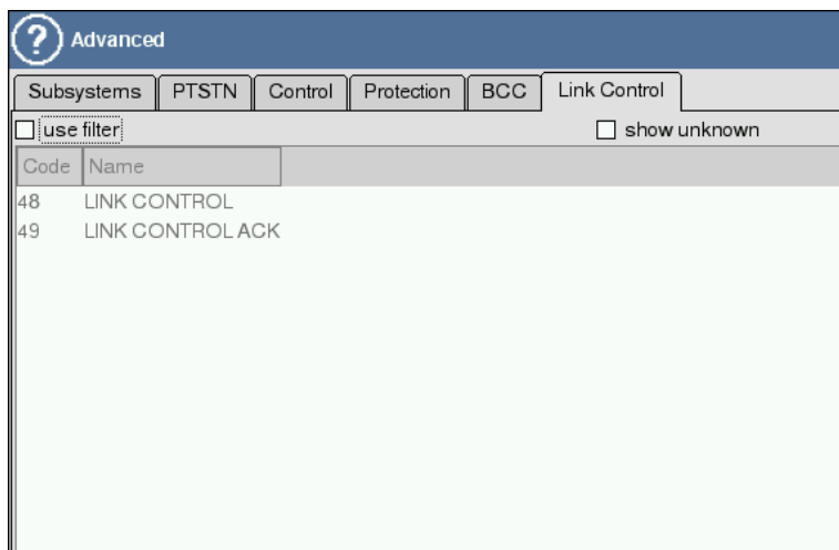
Рис. 5.27. Дополнительная настройка фильтров для V5: Link Control
