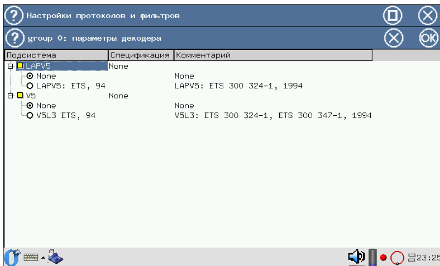
Рис. 5.19. Меню выбора декодера для протокола V5
