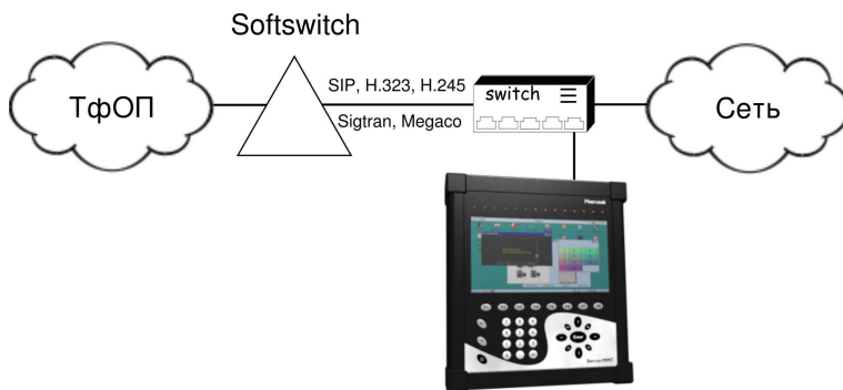
Рис. 3.2. Схема подключения к сети NGN
