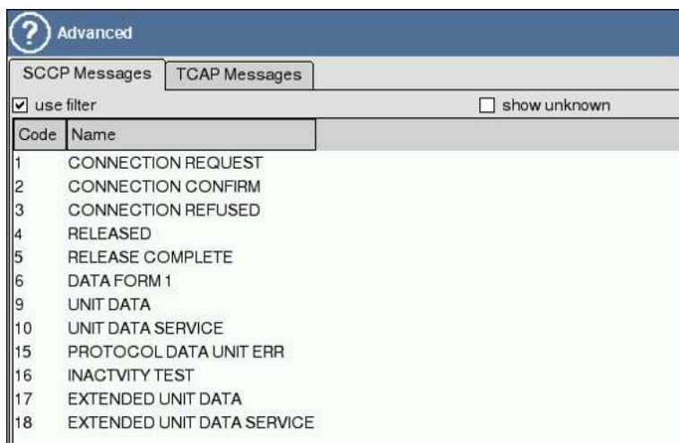
Рис. 5.20. Дополнительные настройки SS7/TCAP: SSCP
