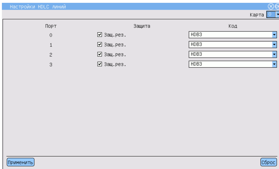
Рис. 4.1. Настройка HDLC-линий
