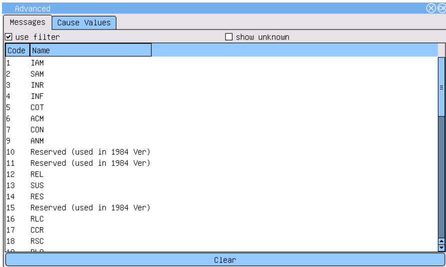
Рис. 5.29. SS7/ISUP, EDSS1/PRI, DSS1/PRI: фильтр по типу сообщения
