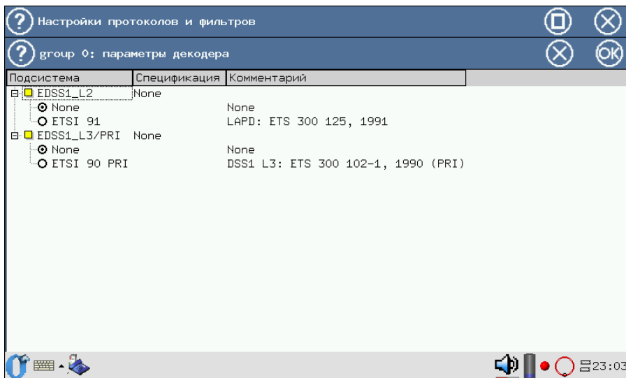
Рис. 5.7. Меню выбора декодера для протокола EDSS1/PRI
