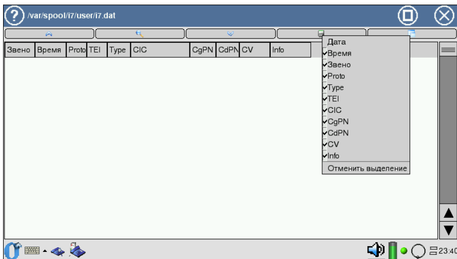
Рис. 6.4. Анализ протоколов DSS1/PRI, EDSS1/PRI
