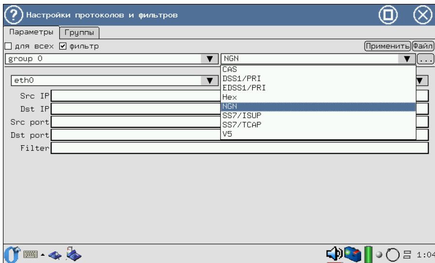
Рис. 4.4. Настройка протоколов и фильтров
