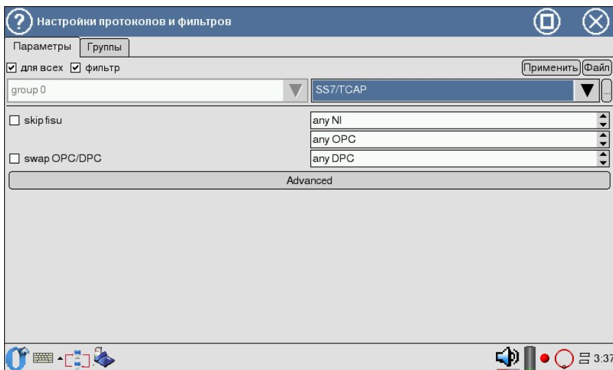
Рис. 5.16. Подсистема фильтров: настройка по протоколам SS7/ТСАР
