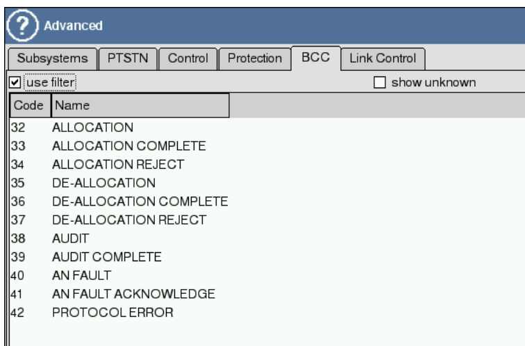
Рис. 5.26. Дополнительная настройка фильтров для V5: BCC
