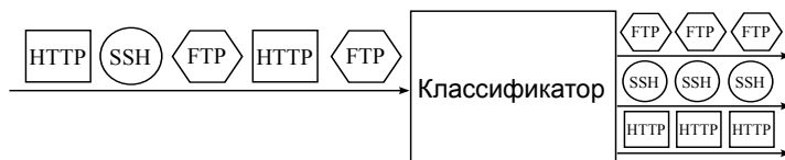
Рис. 6.1. Принцип работы классификатора
