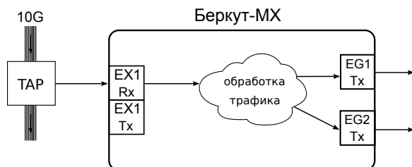
Рис. 7.1. Типовая схема подключения 1
