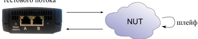
Рис. 11.2. Измерение джиттера. Схема 2
