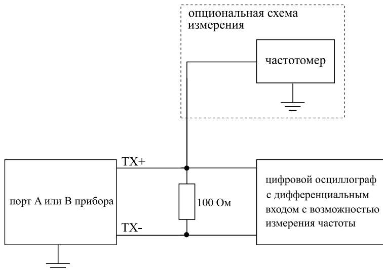
Рис. 16.1. Схема подключения
