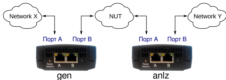
Рис. 8.1. Пример схемы тестирования без влияния на пользовательский трафик
